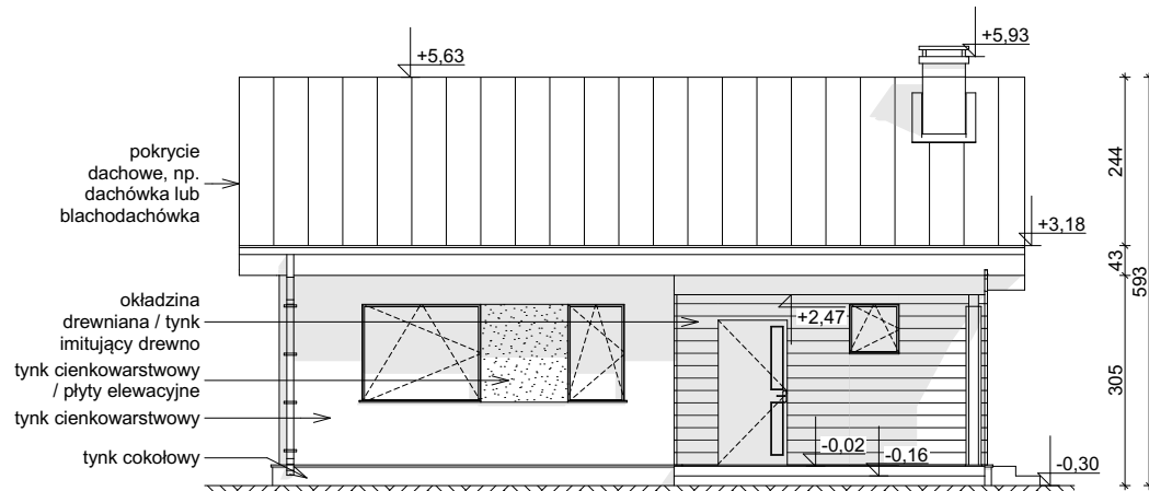
ELEWACJA FRONTOWA
