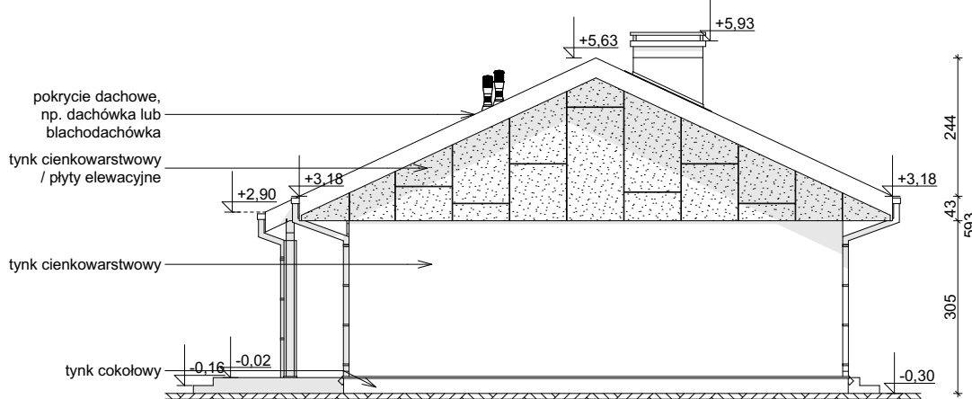
ELEWACJA BOCZNA
