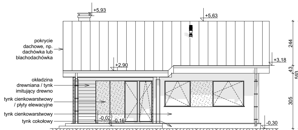
ELEWACJA OGRODOWA
