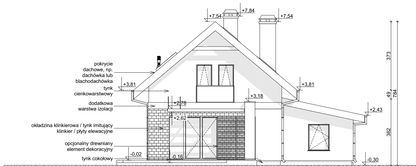
ELEWACJA OGRODOWA
