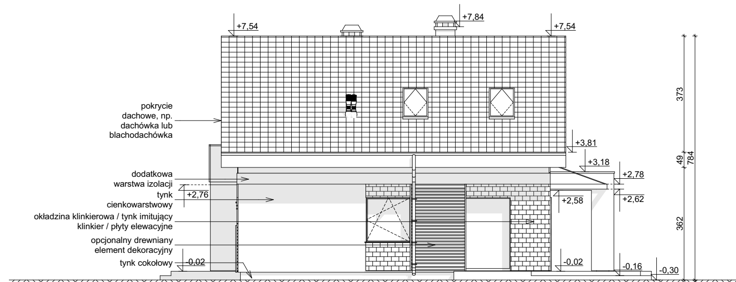
ELEWACJA BOCZNA
