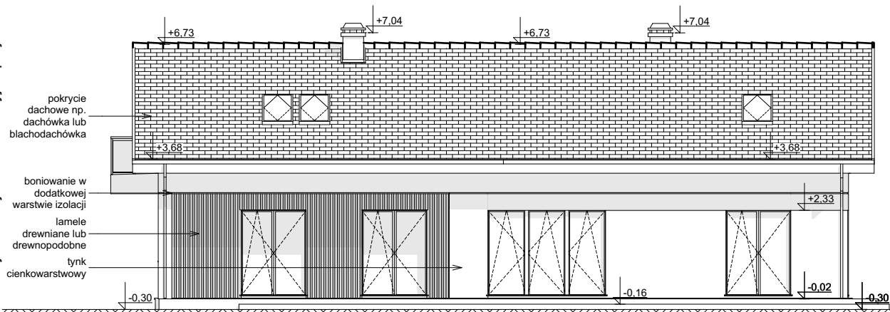
ELEWACJA OGRODOWA
