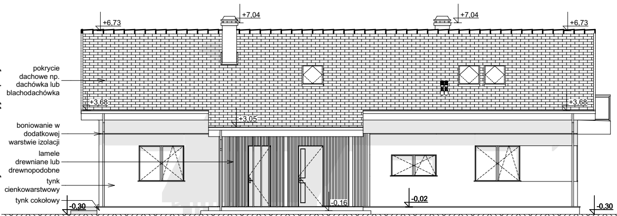
ELEWACJA FRONTOWA
