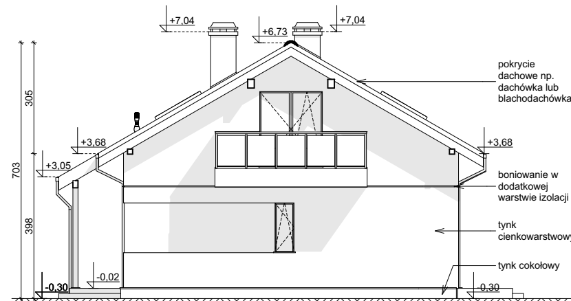
ELEWACJA BOCZNA
