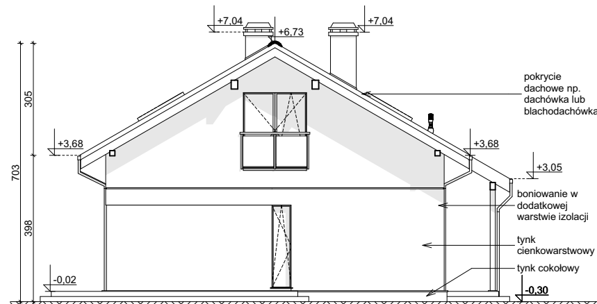
ELEWACJA BOCZNA
