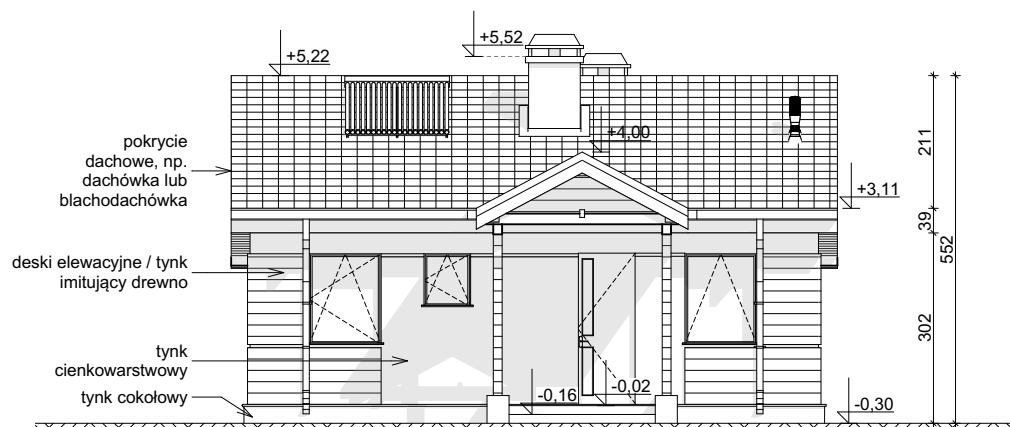
ELEWACJA FRONTOWA
