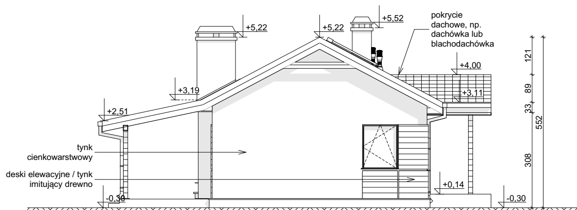
ELEWACJA BOCZNA
