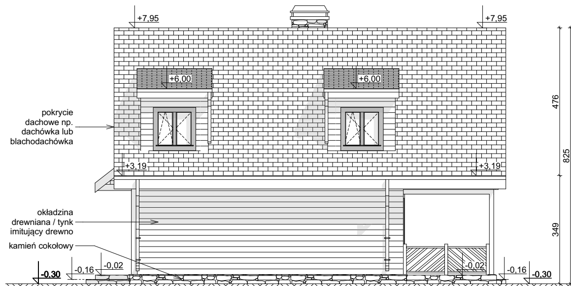
ELEWACJA BOCZNA
