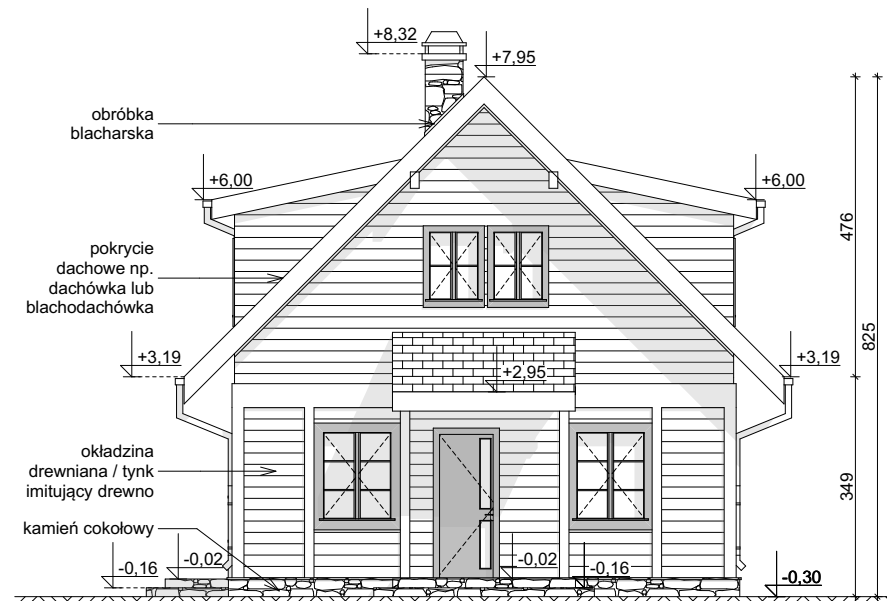
ELEWACJA FRONTOWA
