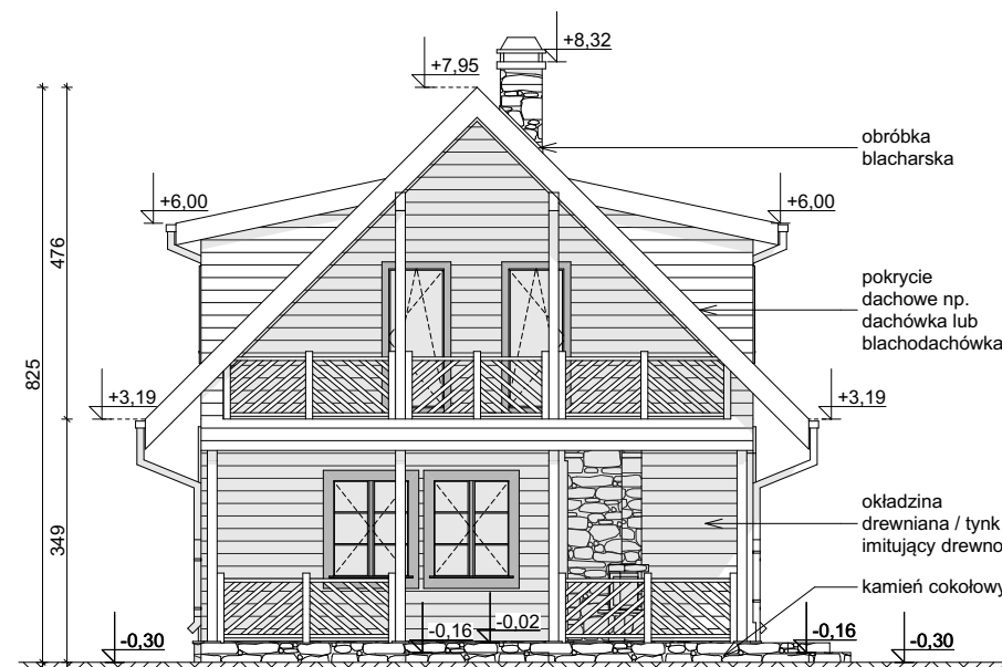
ELEWACJA OGRODOWA
