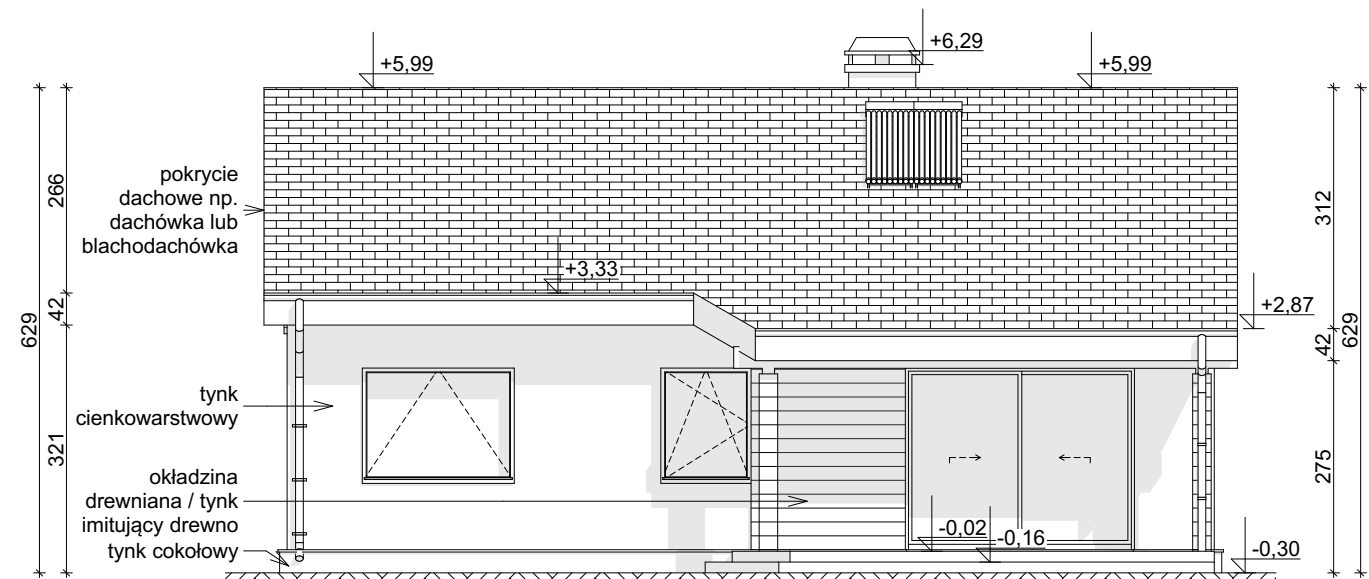
ELEWACJA OGRODOWA
