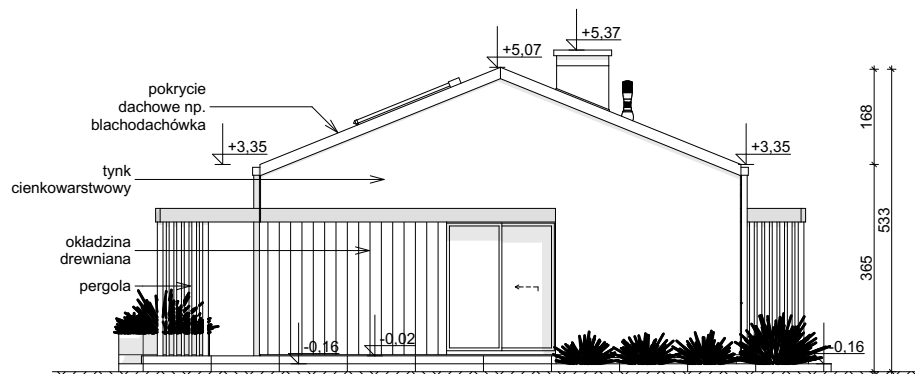
ELEWACJA BOCZNA
