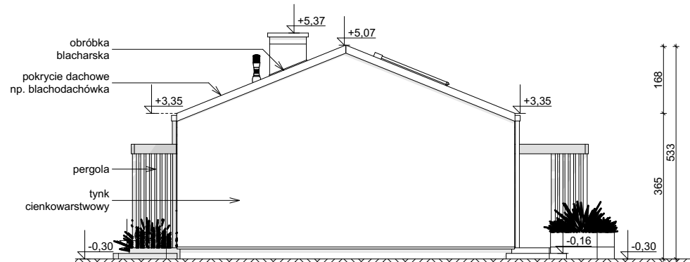
ELEWACJA BOCZNA
