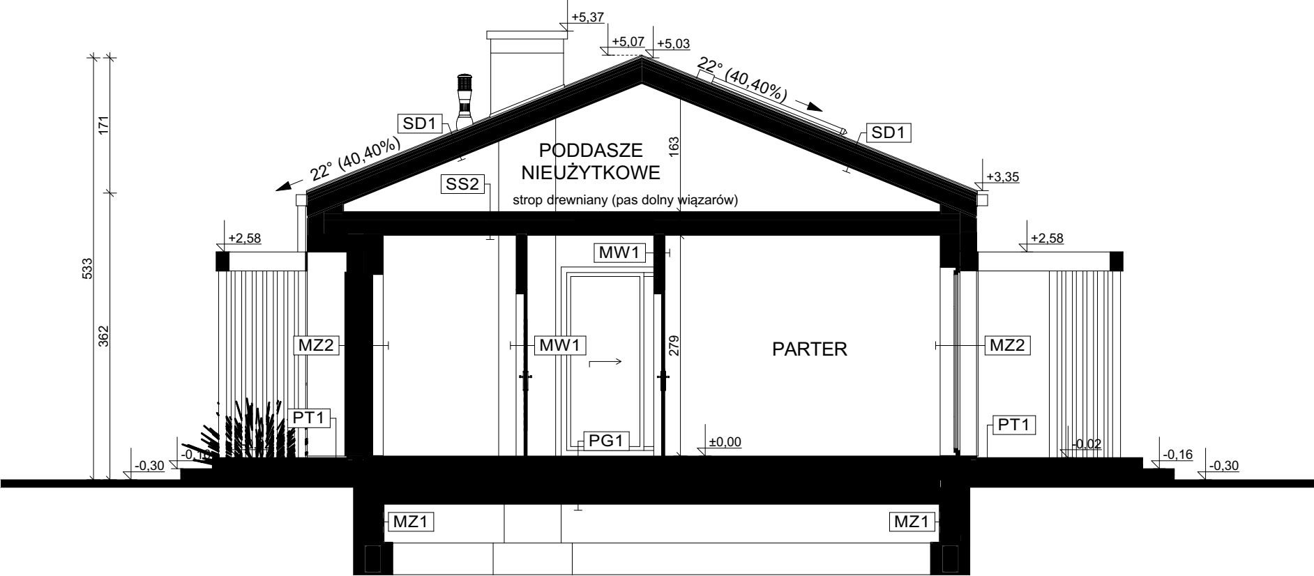
PRZEKRÓJ B-B
