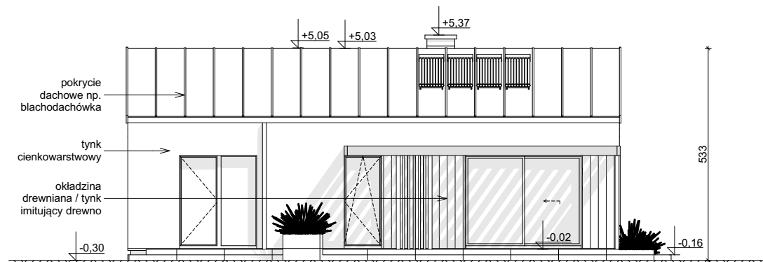
ELEWACJA OGRODOWA
