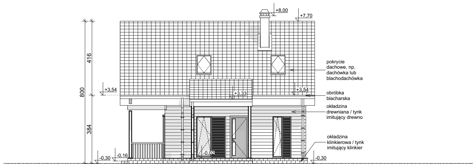
ELEWACJA FRONTOWA
