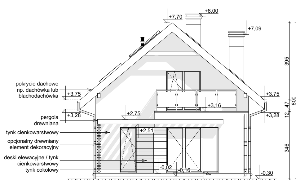
ELEWACJA OGRODOWA
