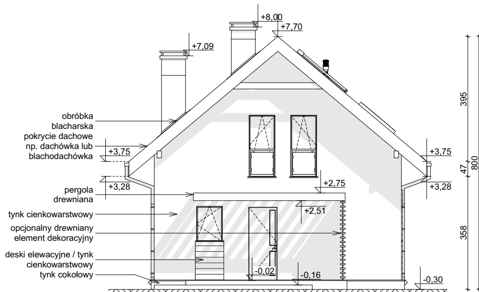
ELEWACJA FRONTOWA
