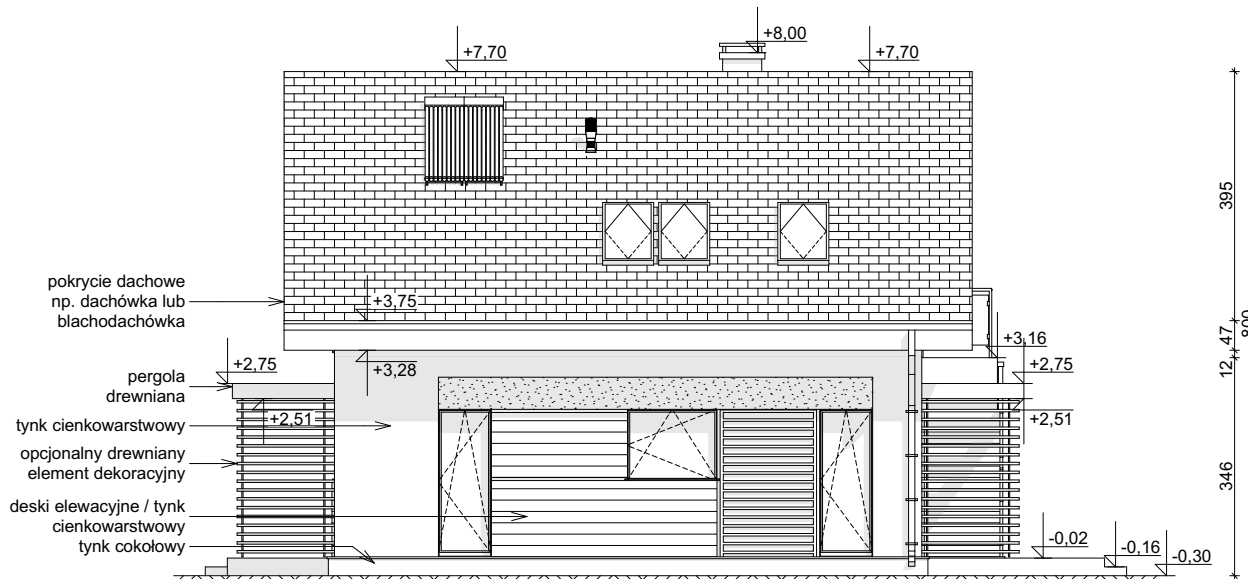
ELEWACJA BOCZNA
