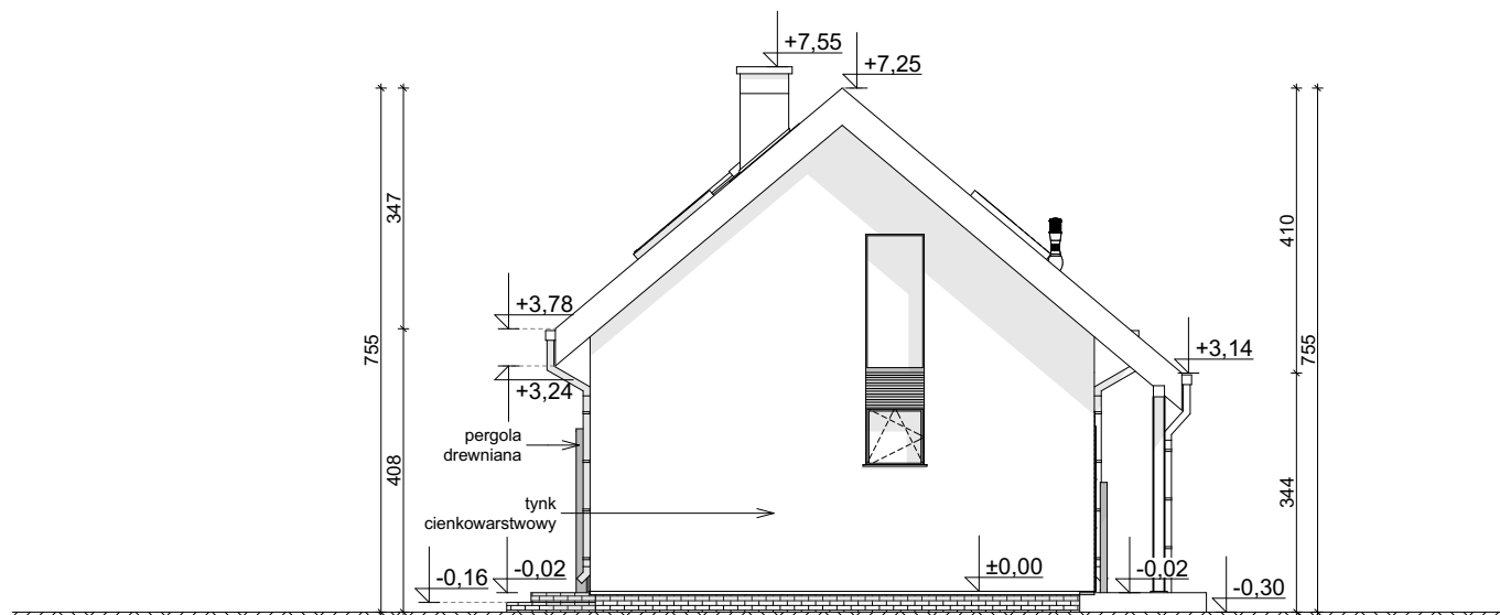
ELEWACJA BOCZNA
