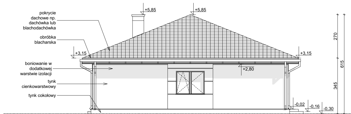
ELEWACJA BOCZNA
