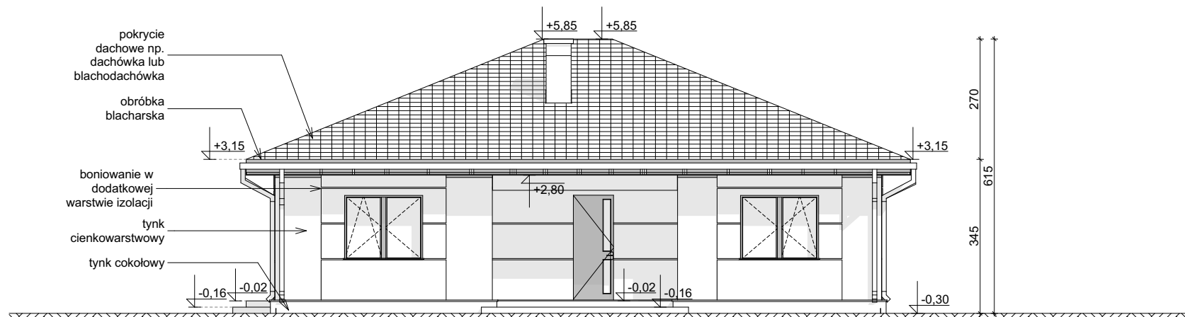
ELEWACJA FRONTOWA
