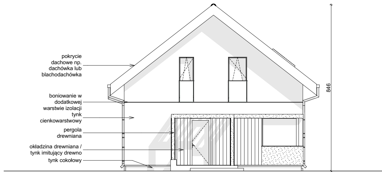
ELEWACJA FRONTOWA
