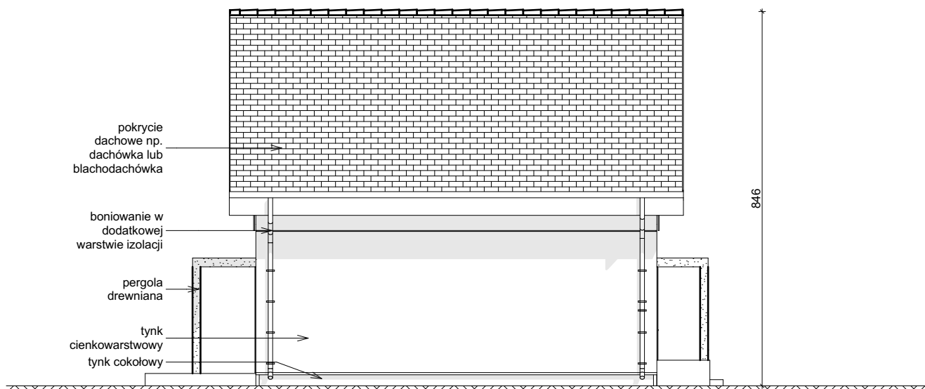
ELEWACJA BOCZNA
