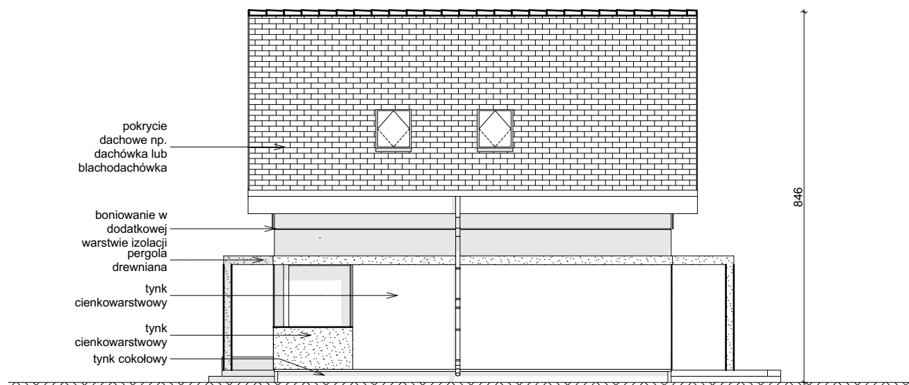
ELEWACJA BOCZNA
