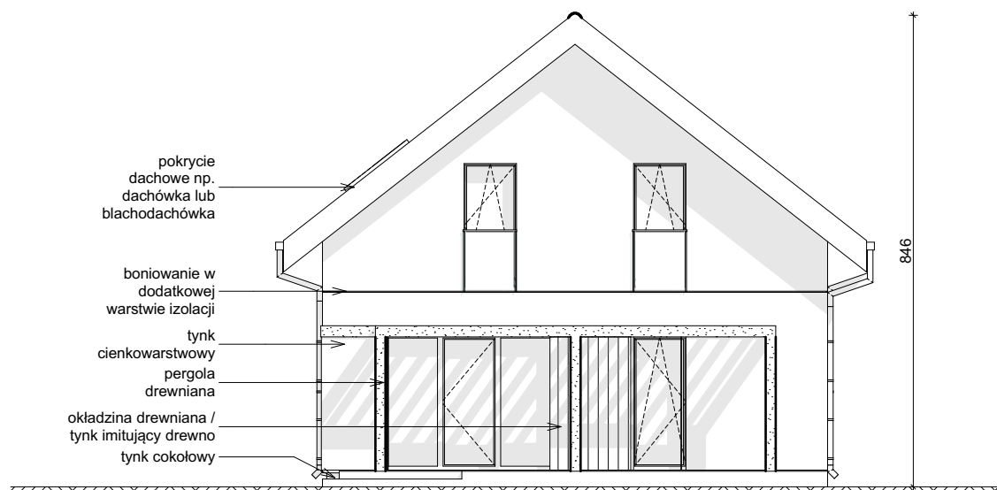
ELEWACJA OGRODOWA
