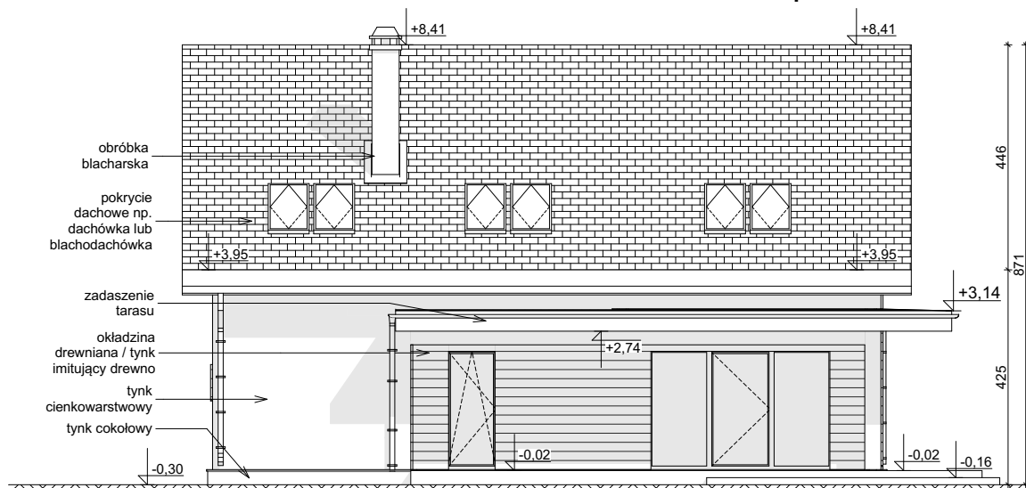
ELEWACJA OGRODOWA
