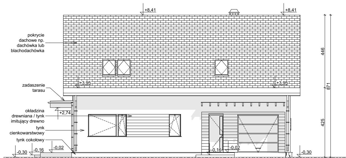
ELEWACJA FRONTOWA
