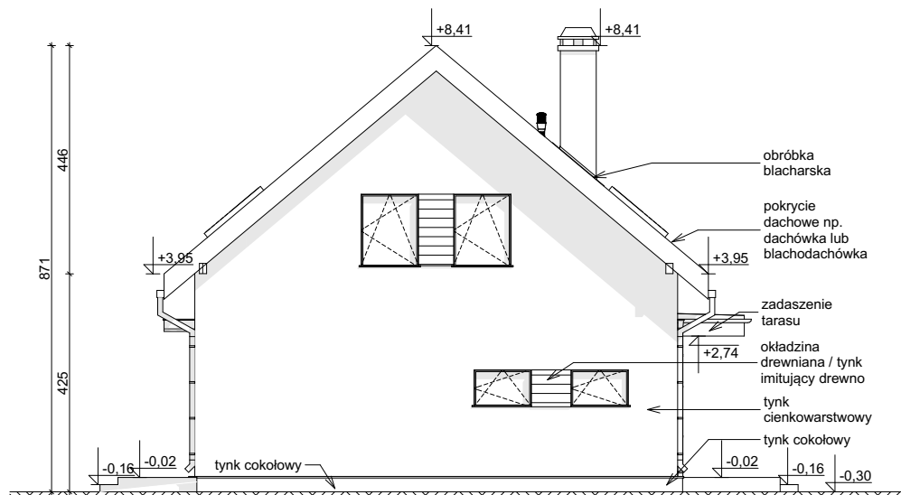
ELEWACJA BOCZNA
