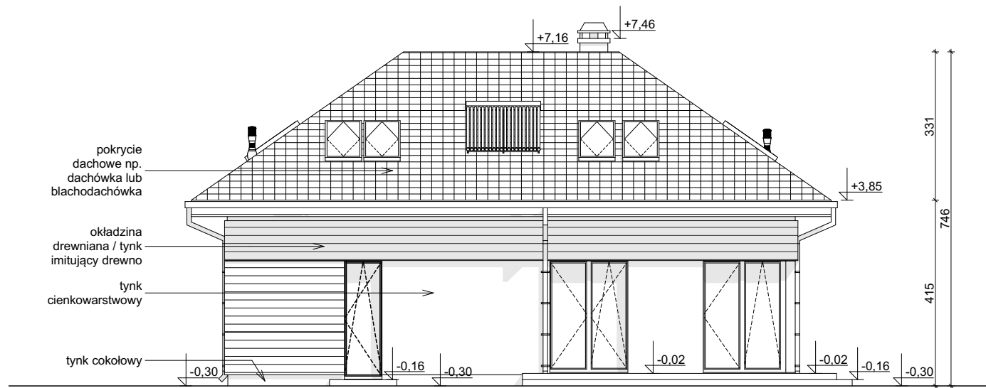
ELEWACJA OGRODOWA
