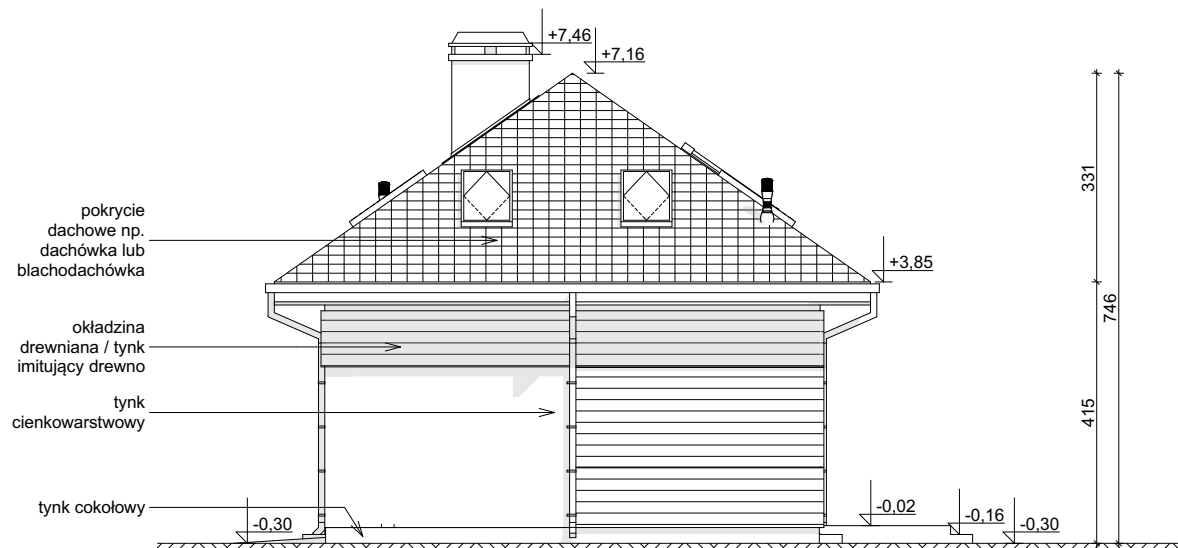
ELEWACJA BOCZNA
