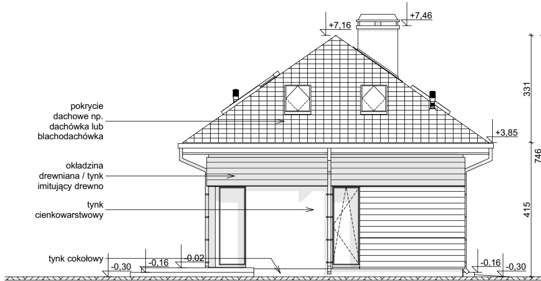
ELEWACJA BOCZNA
