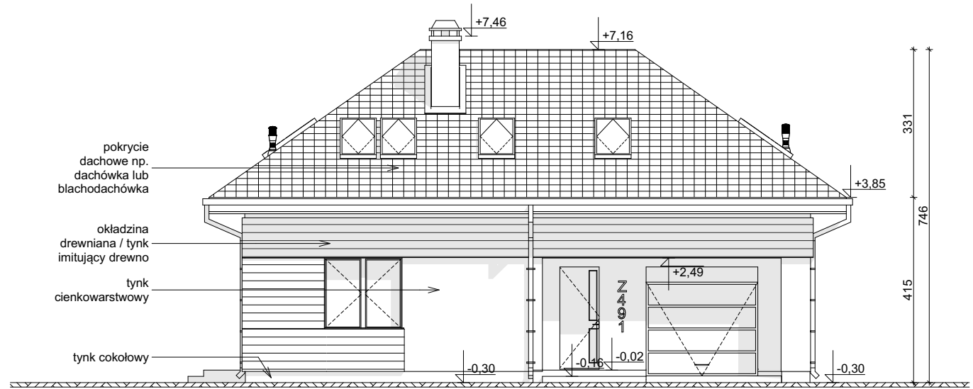
ELEWACJA FRONTOWA
