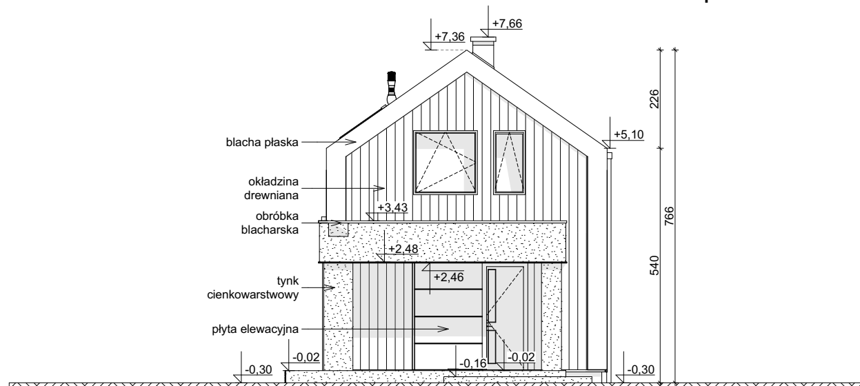
ELEWACJA FRONTOWA
