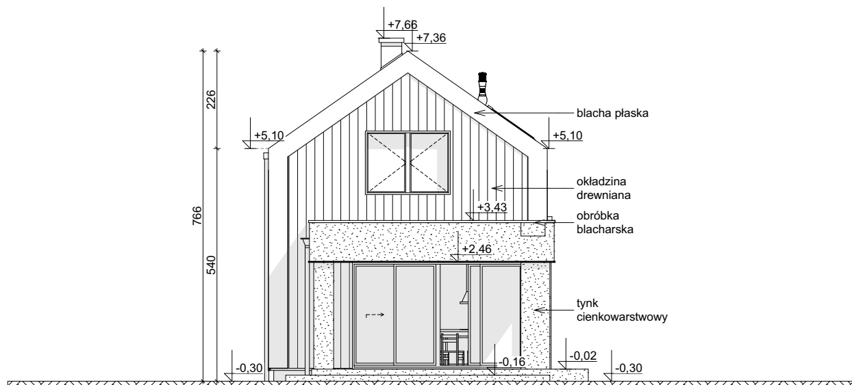
ELEWACJA OGRODOWA
