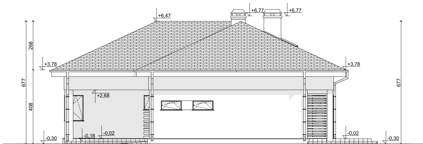
ELEWACJA BOCZNA
