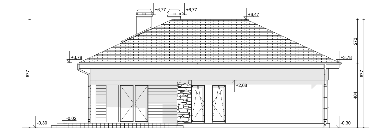
ELEWACJA BOCZNA
