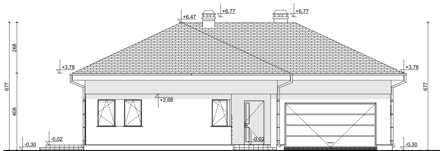
ELEWACJA FRONTOWA
