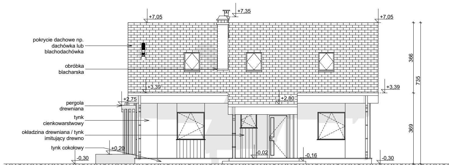
ELEWACJA FRONTOWA
