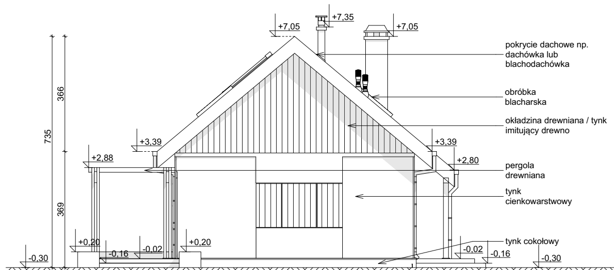
ELEWACJA BOCZNA
