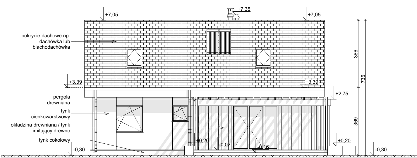
ELEWACJA OGRODOWA
