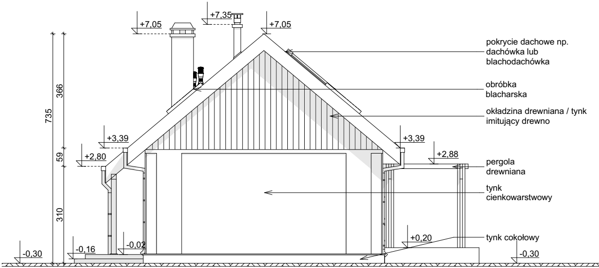
ELEWACJA BOCZNA
