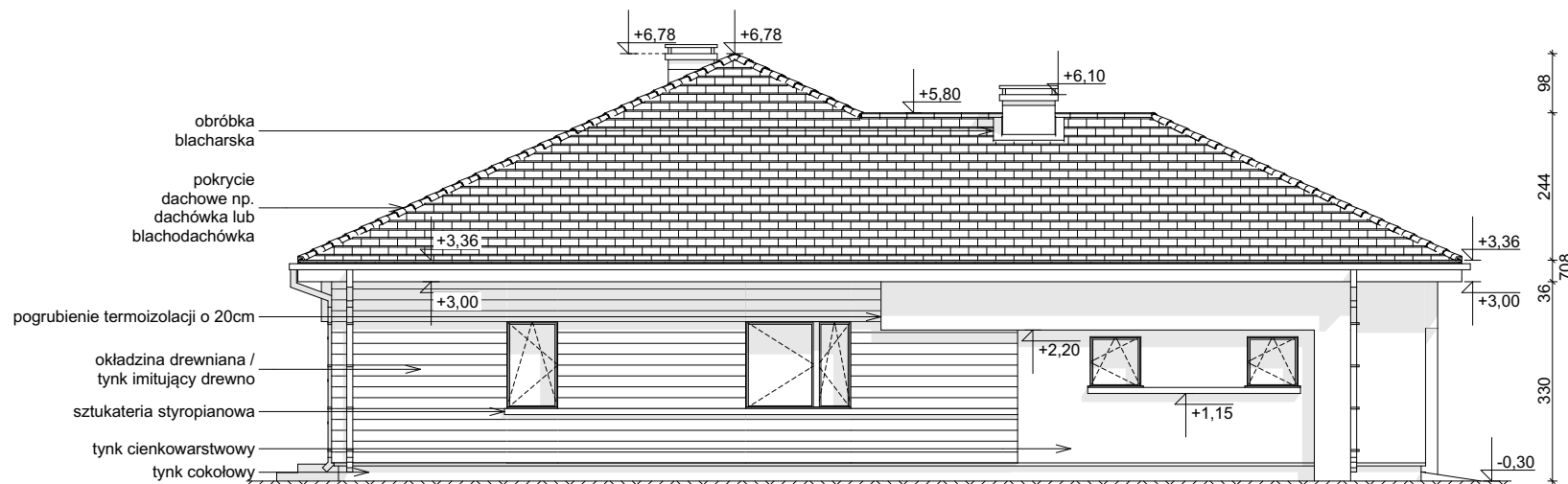
ELEWACJA BOCZNA
