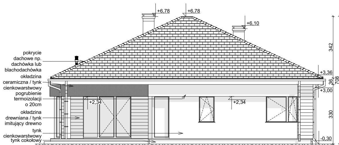
ELEWACJA OGRODOWA
