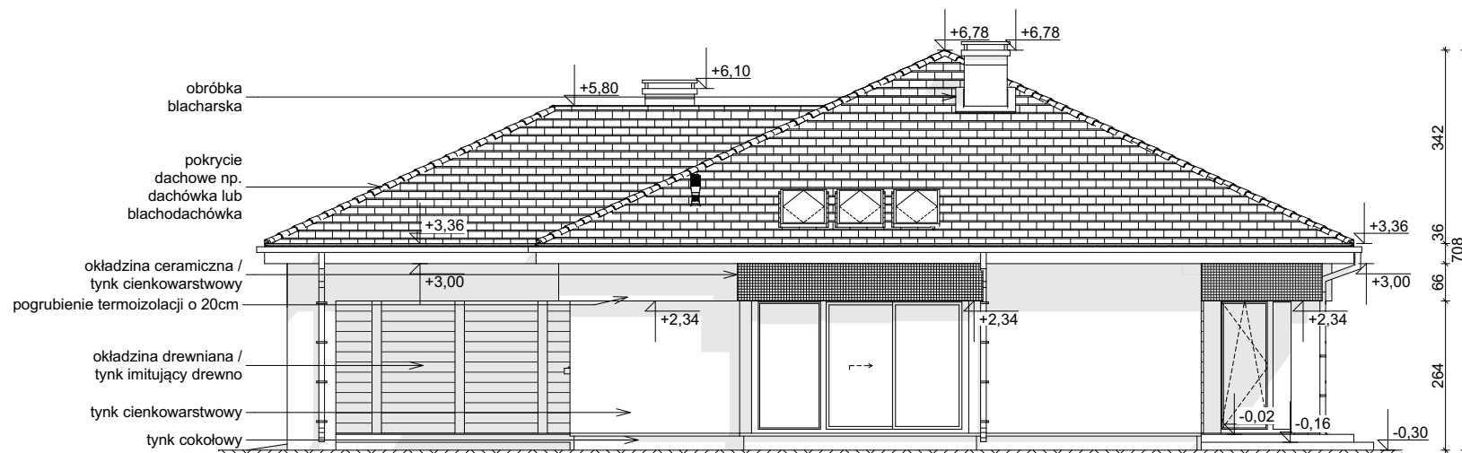
ELEWACJA BOCZNA
