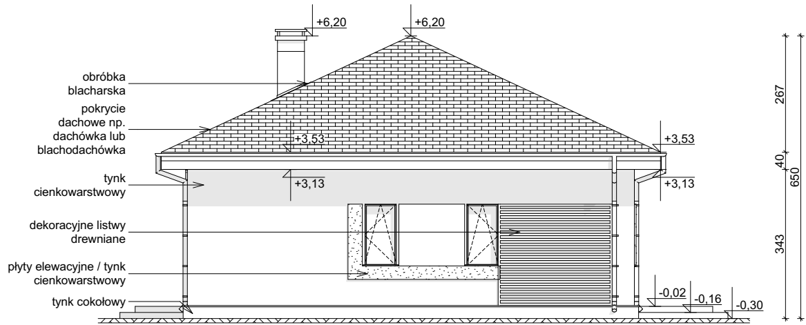
ELEWACJA BOCZNA
