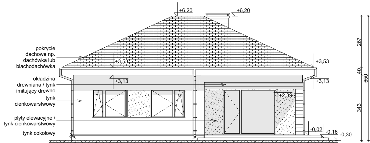
ELEWACJA OGRODOWA
