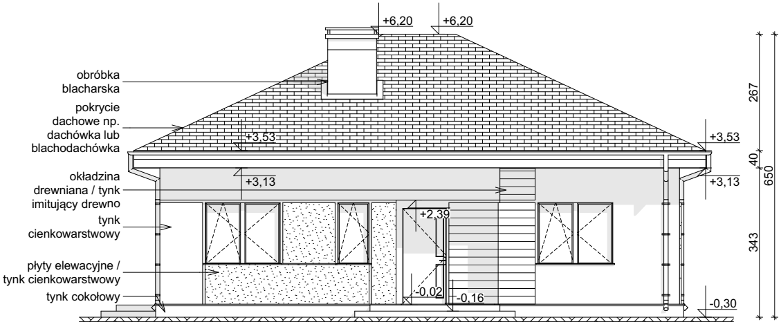
ELEWACJA FRONTOWA
