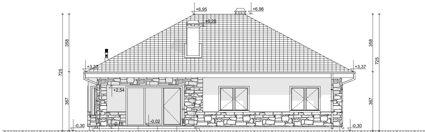
ELEWACJA BOCZNA
