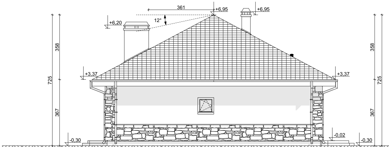
ELEWACJA BOCZNA
