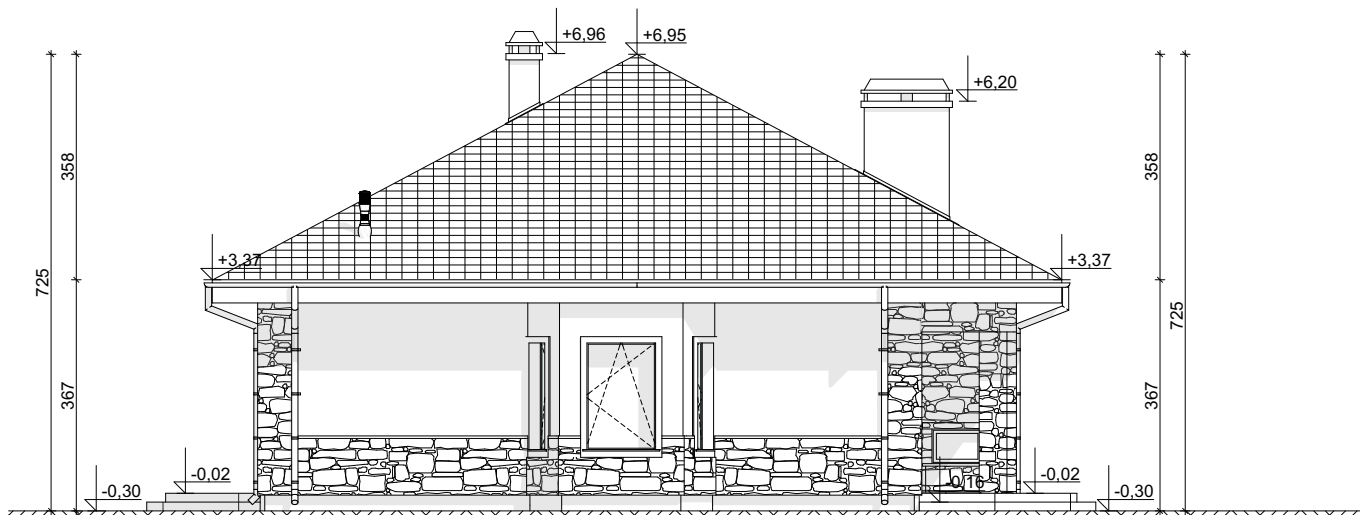
ELEWACJA BOCZNA
