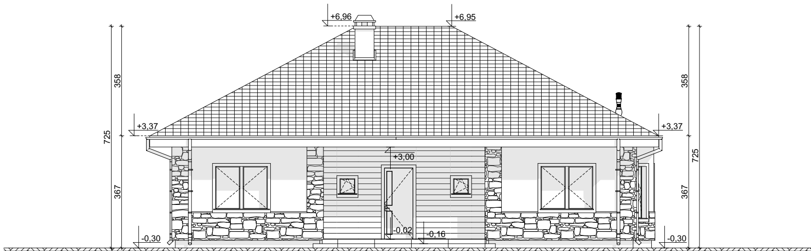
ELEWACJA FRONTOWA
