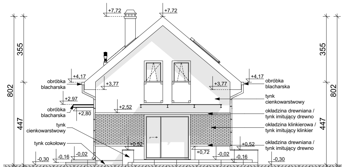
ELEWACJA BOCZNA
