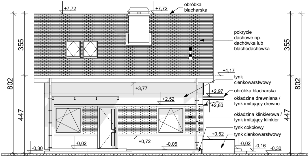
ELEWACJA FRONTOWA
