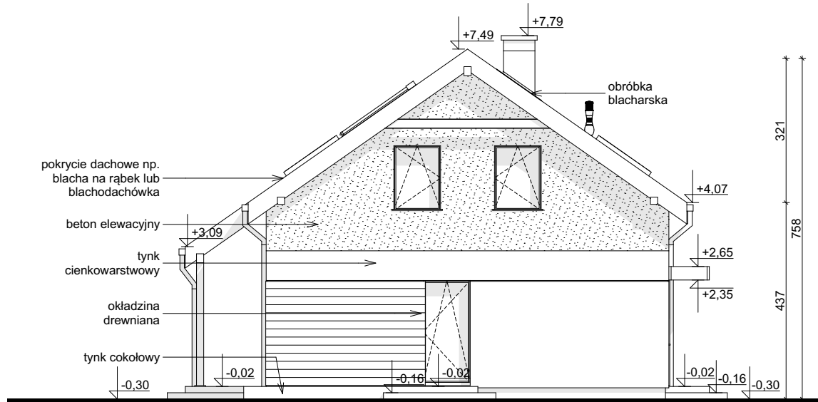
ELEWACJA BOCZNA
