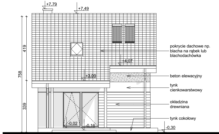
ELEVACJA OGRODOWA
