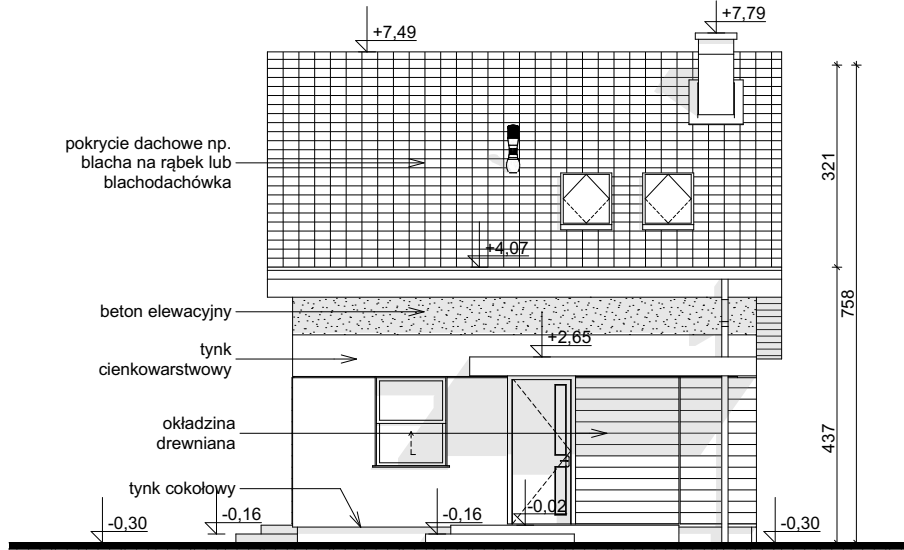
ELEWACJA FRONTOWA
