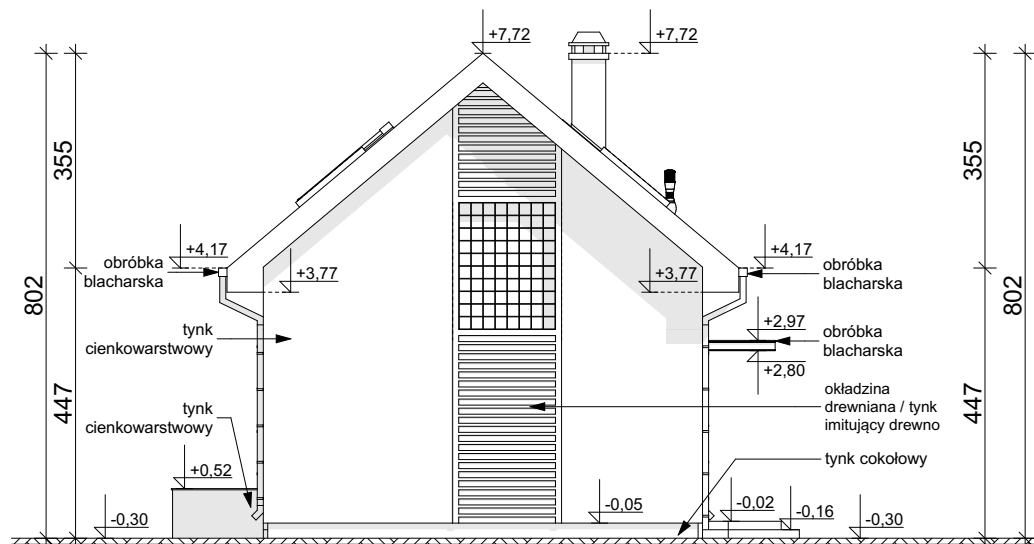
ELEWACJA BOCZNA
