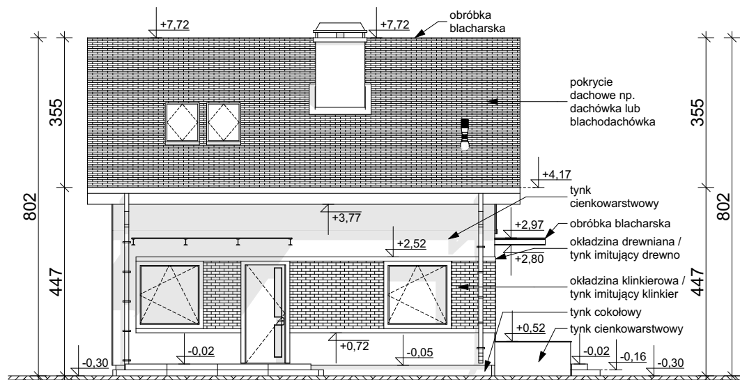
ELEWACJA FRONTOWA
