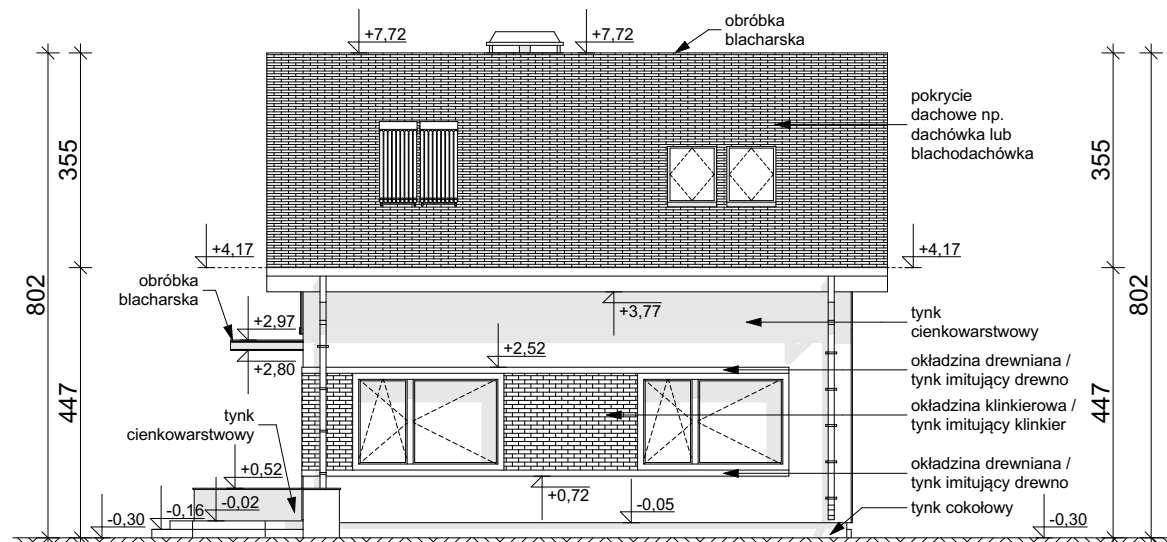
ELEWACJA OGRODOWA
