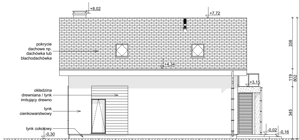
ELEWACJA OGRODOWA
