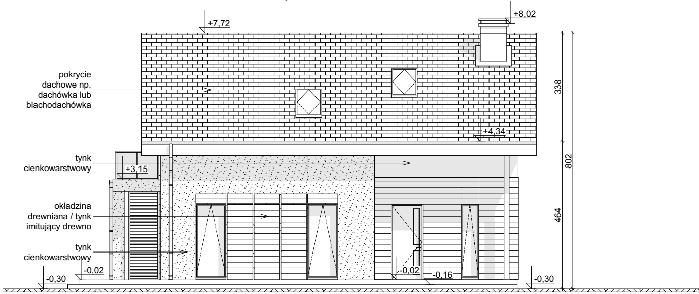
ELEWACJA FRONTOWA
