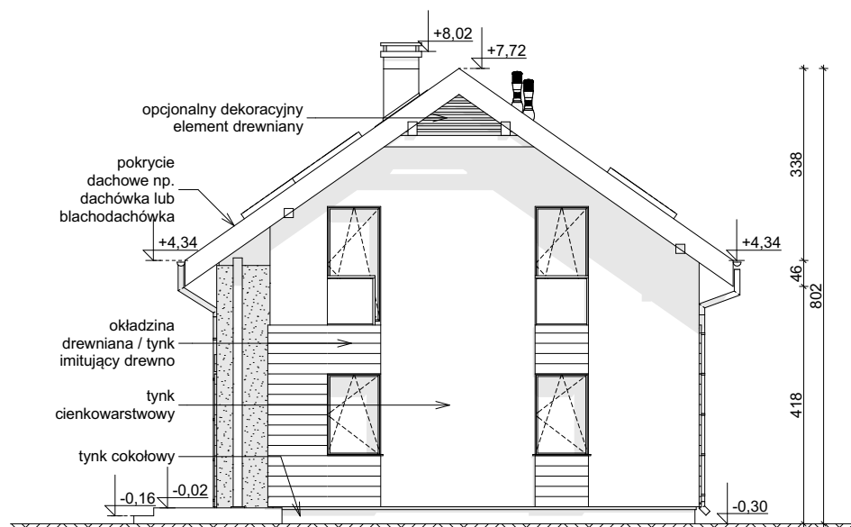
ELEWACJA BOCZNA
