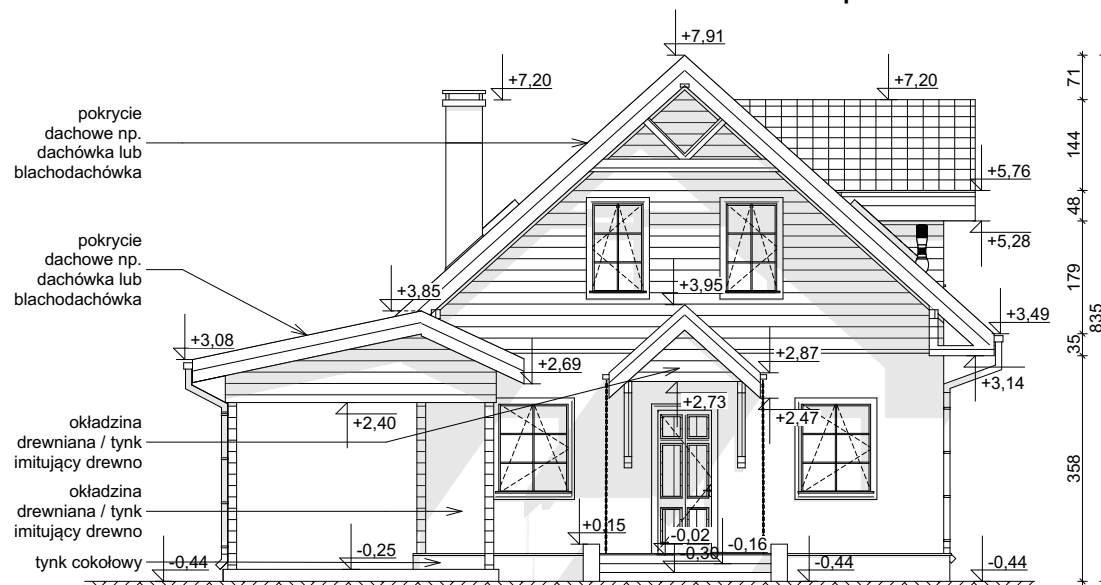
ELEWACJA FRONTOWA
