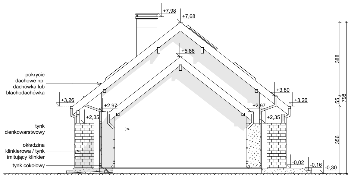
ELEWACJA BOCZNA
