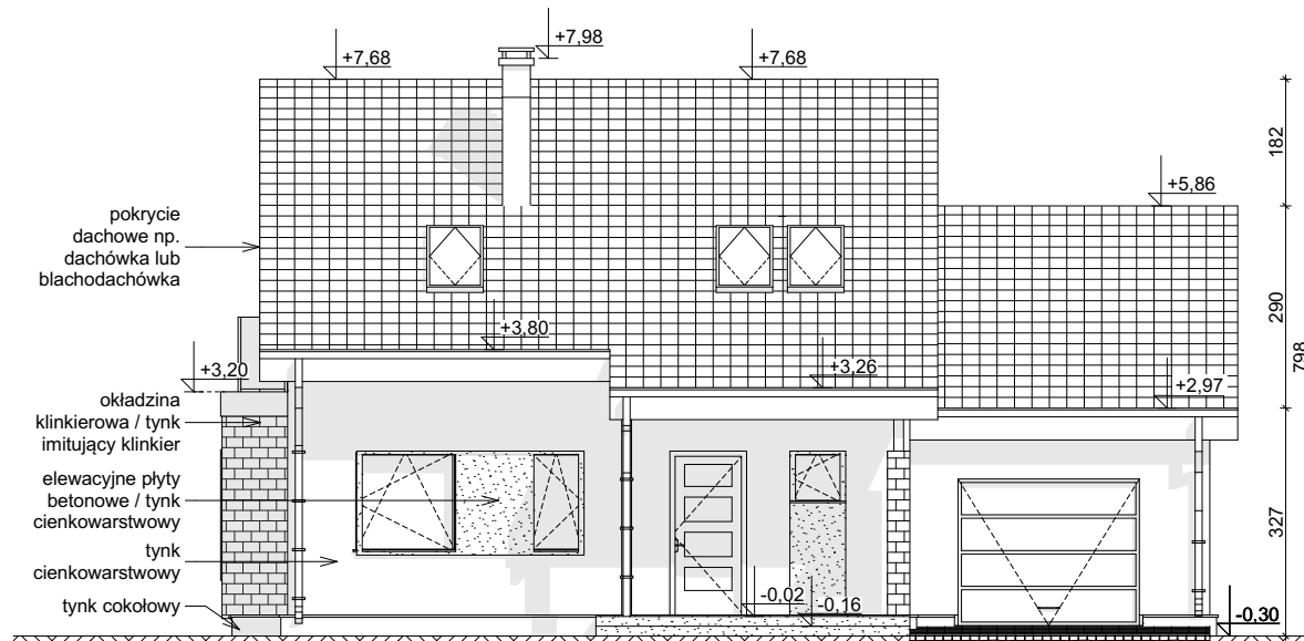
ELEWACJA FRONTOWA
