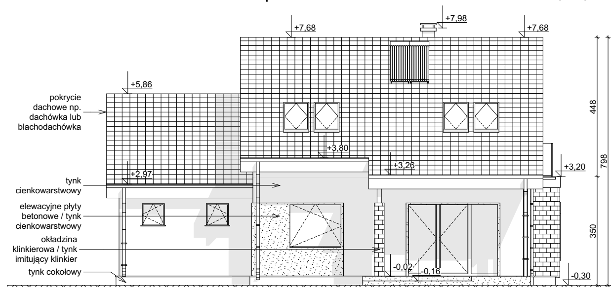
ELEWACJA OGRODOWA
