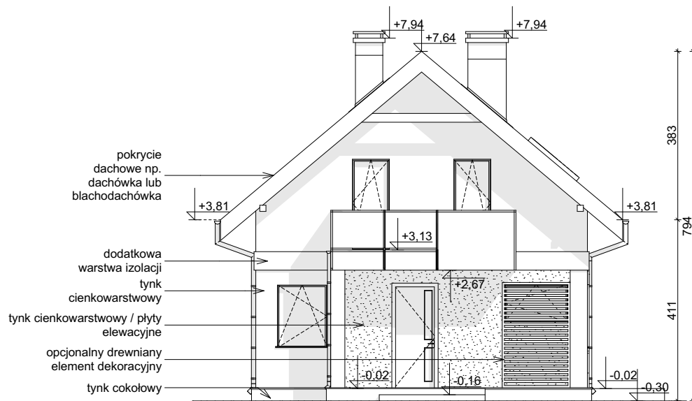
ELEWACJA FRONTOWA
