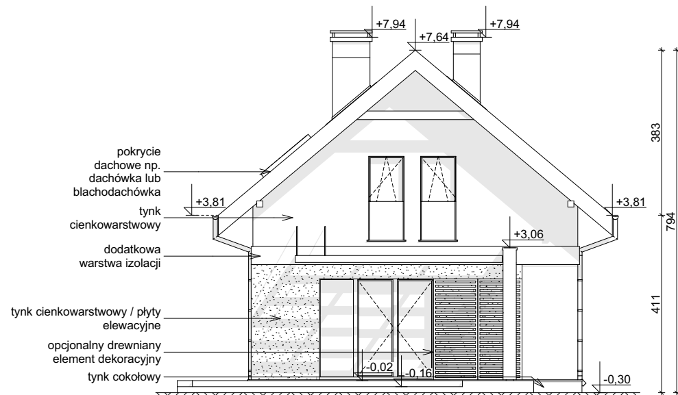
ELEWACJA OGRODOWA
