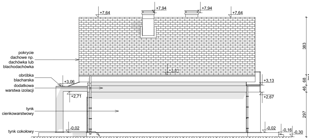
ELEWACJA BOCZNA
