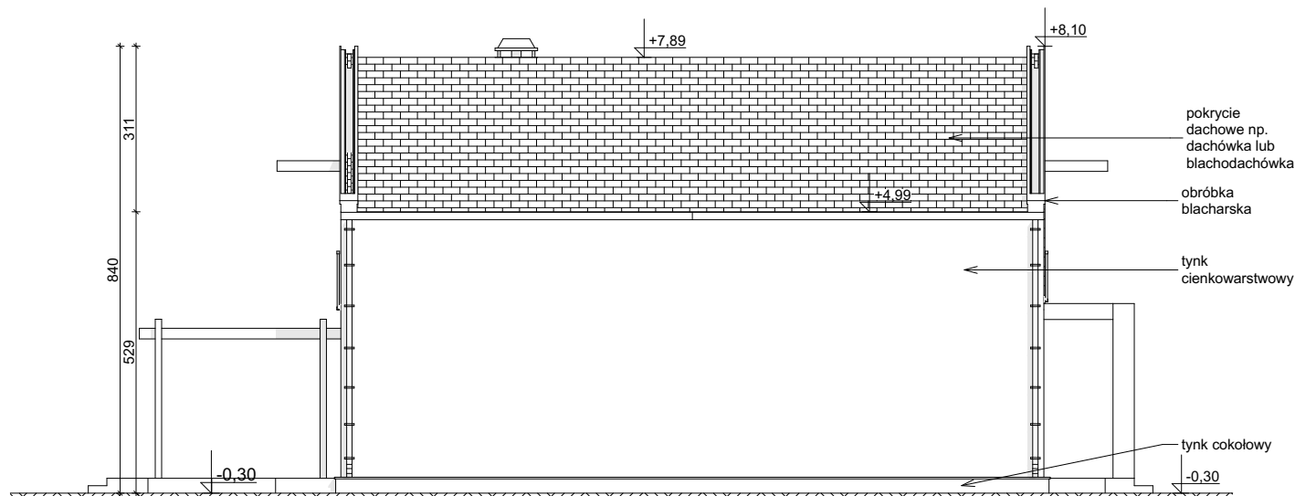
ELEWACJA BOCZNA
