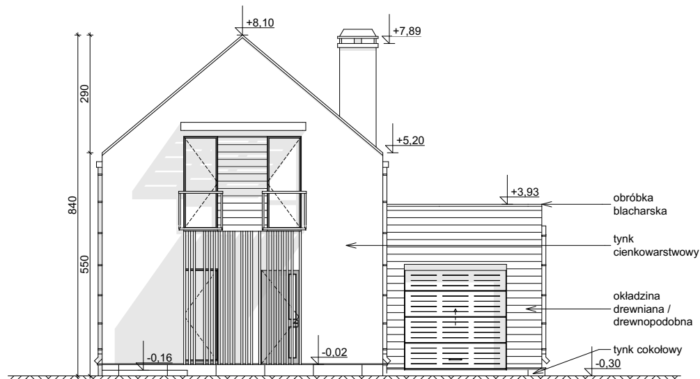
ELEWACJA FRONTOWA
