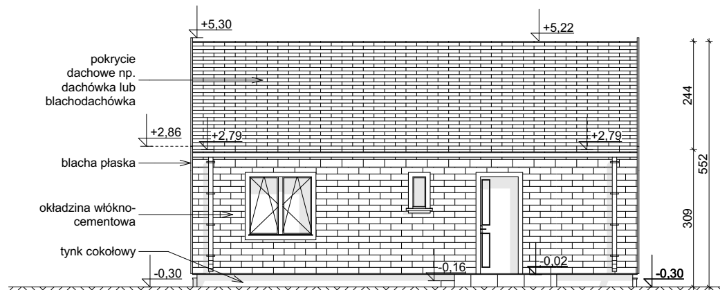
ELEWACJA FRONTOWA
