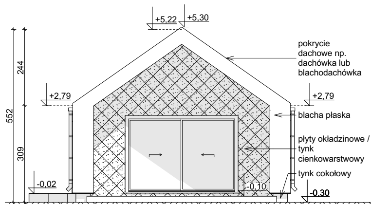
ELEWACJA BOCZNA
