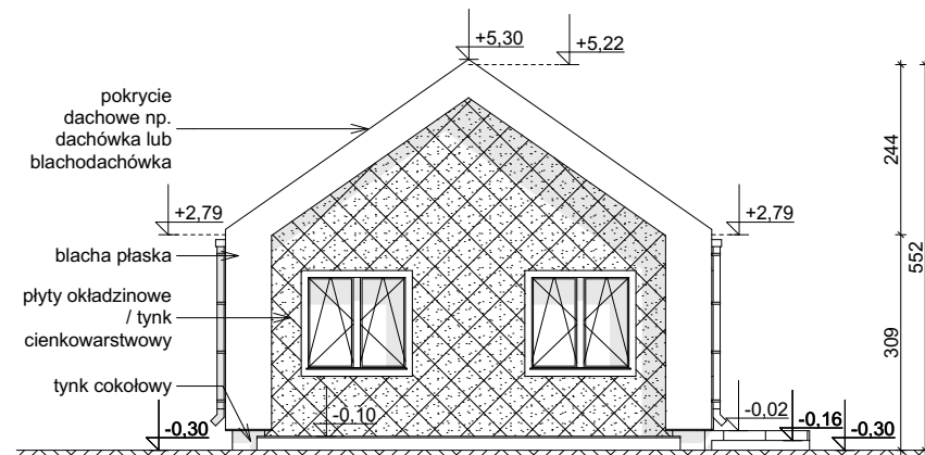
ELEWACJA BOCZNA
