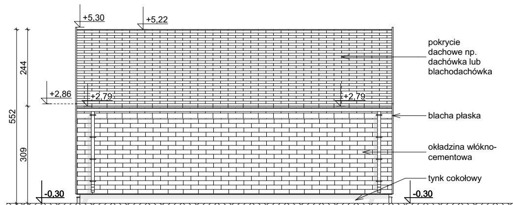
ELEWACJA OGRODOWA
