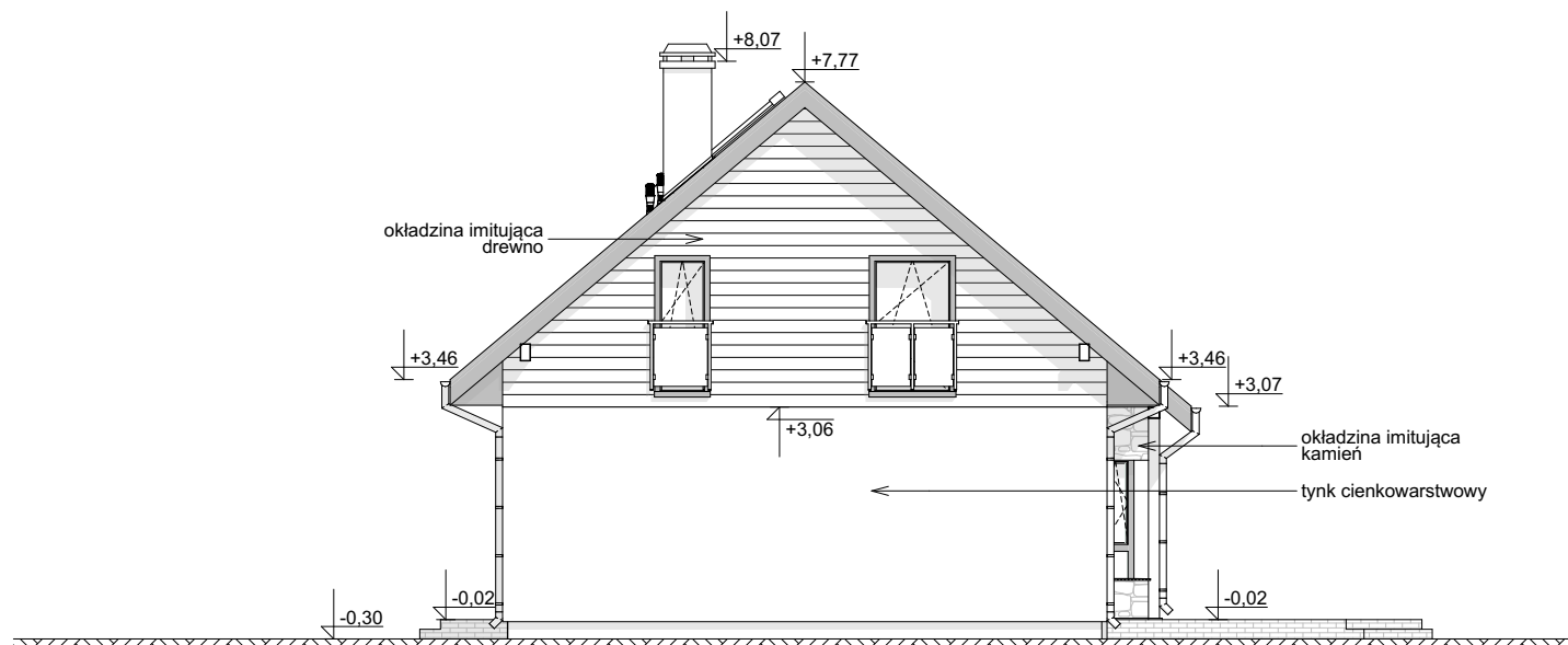
ELEWACJA BOCZNA
