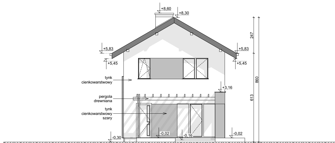
ELEWACJA OGRODOWA
