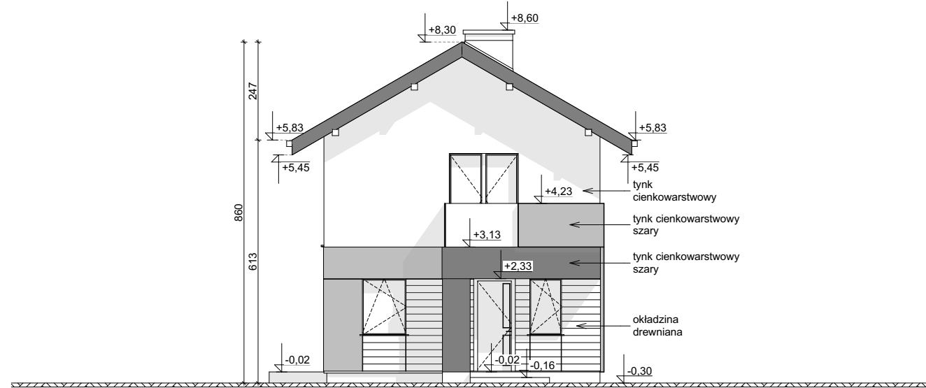
ELEWACJA FRONTOWA
