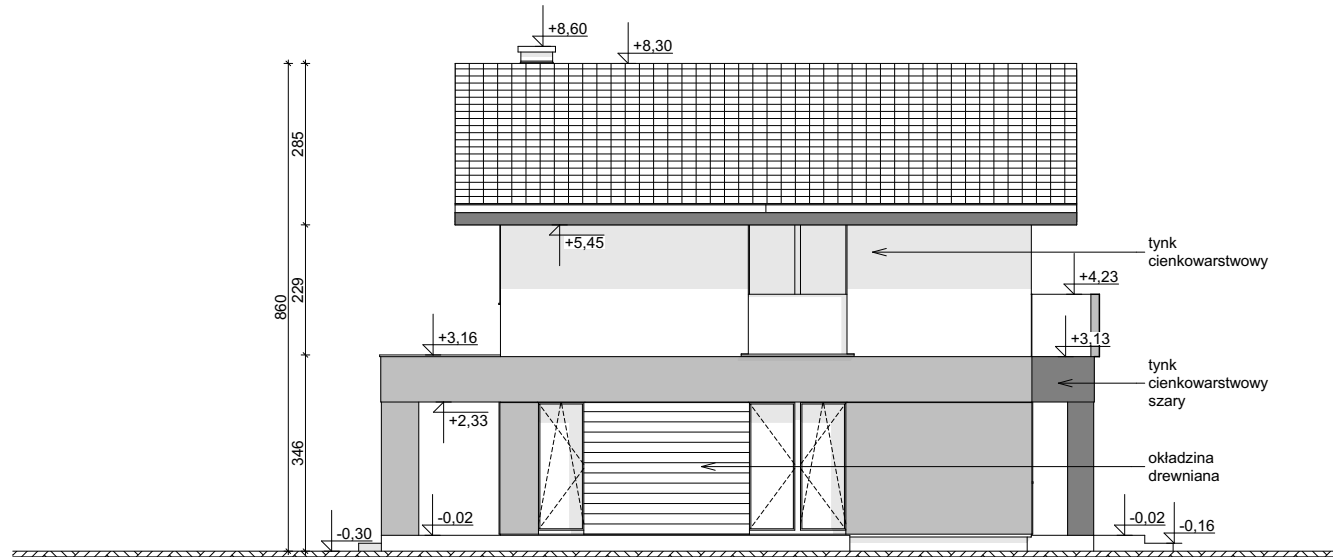
ELEWACJA BOCZNA
