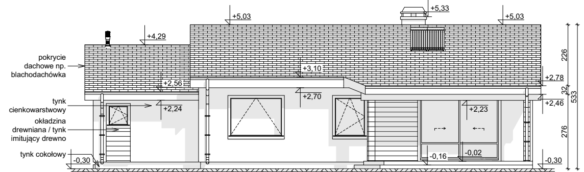
ELEWACJA OGRODOWA
