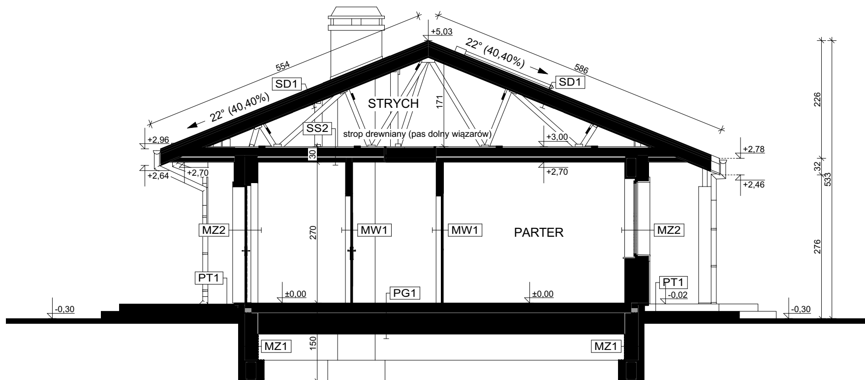
PRZEKRÓJ B-B
