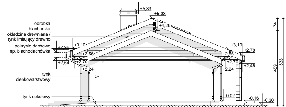
ELEWACJA BOCZNA
