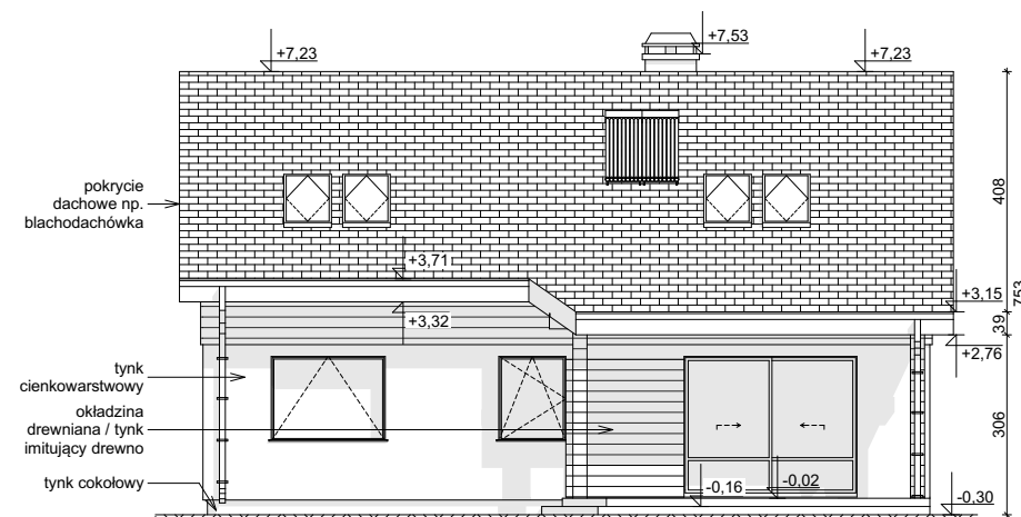
ELEWACJA OGRODOWA
