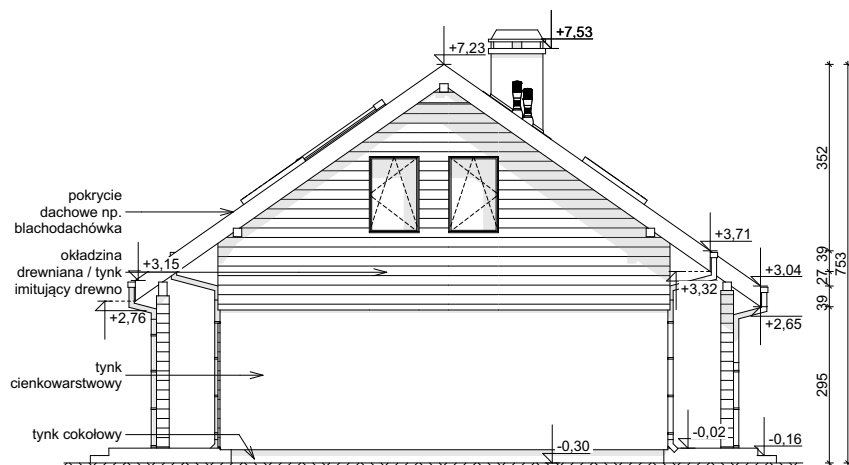
ELEWACJA BOCZNA
