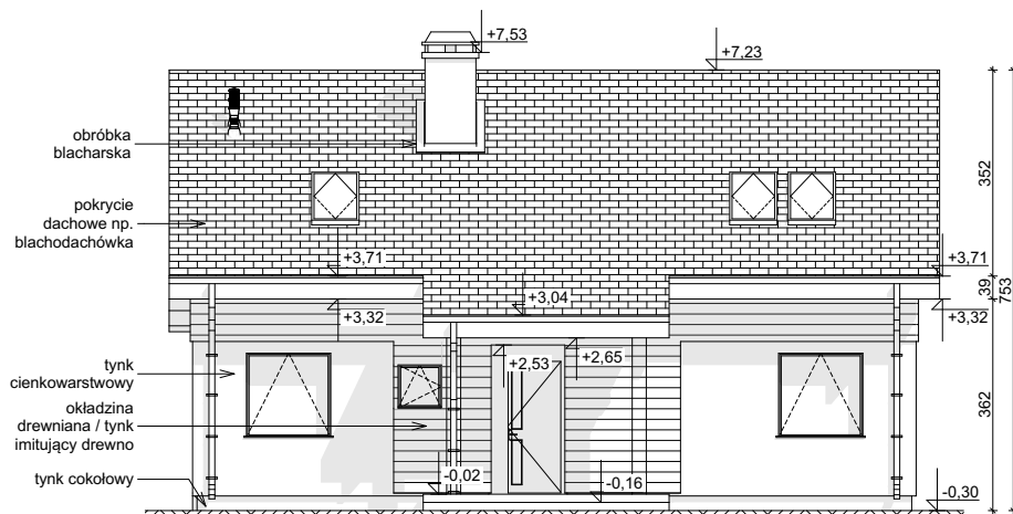
ELEWACJA FRONTOWA
