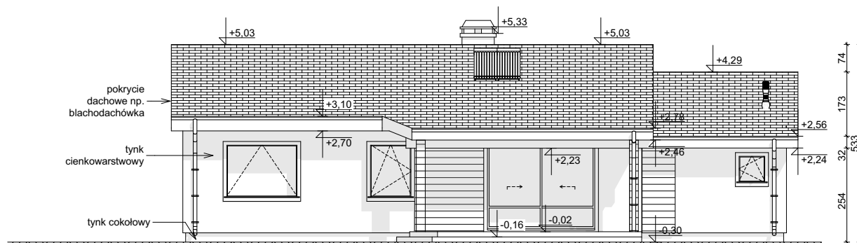
ELEWACJA OGRODOWA
