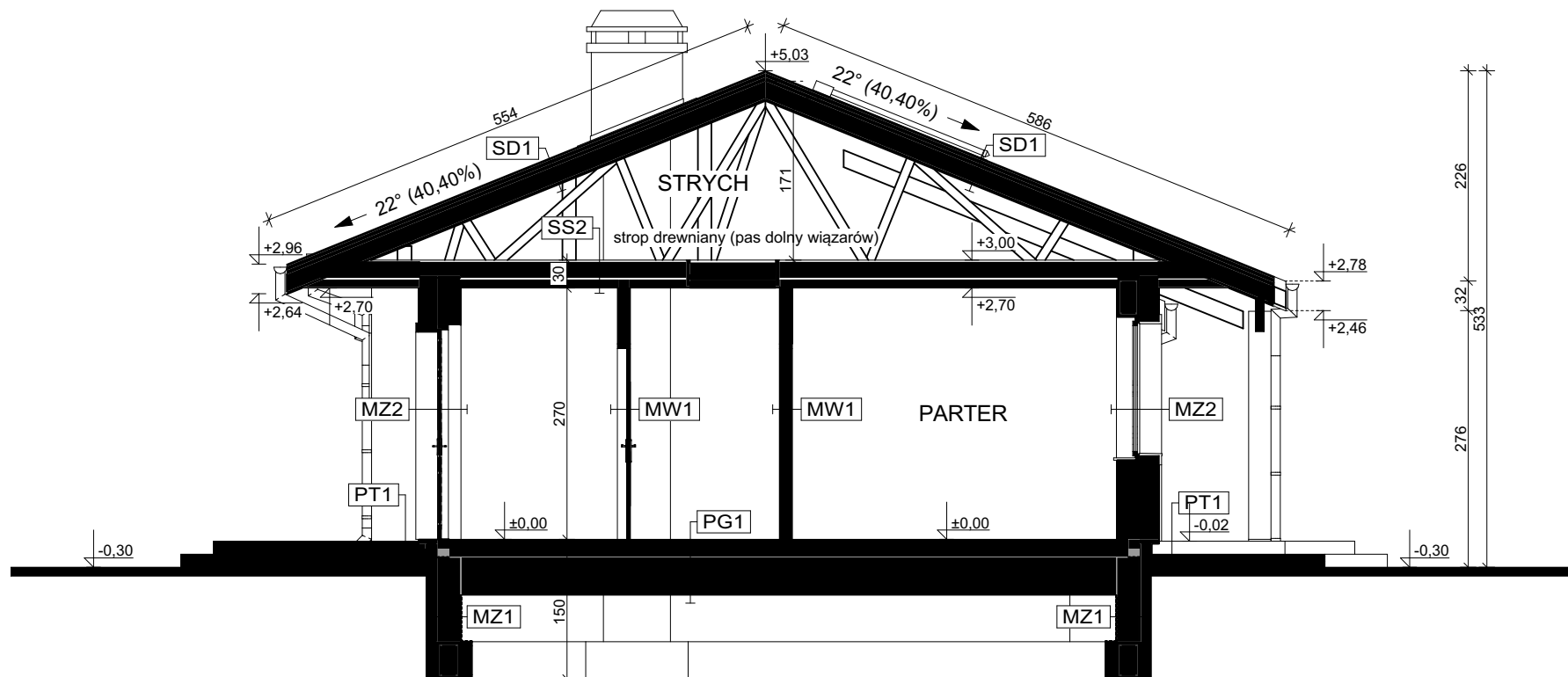
PRZEKRÓJ B-B
