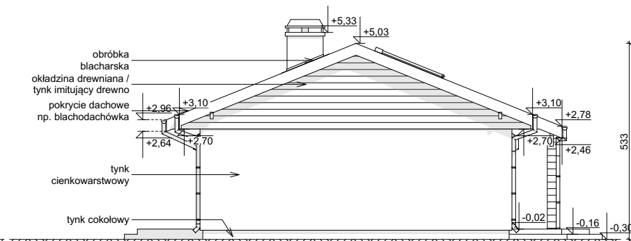
ELEWACJA BOCZNA
