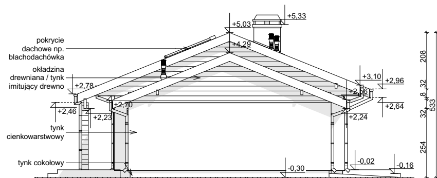
ELEWACJA BOCZNA
