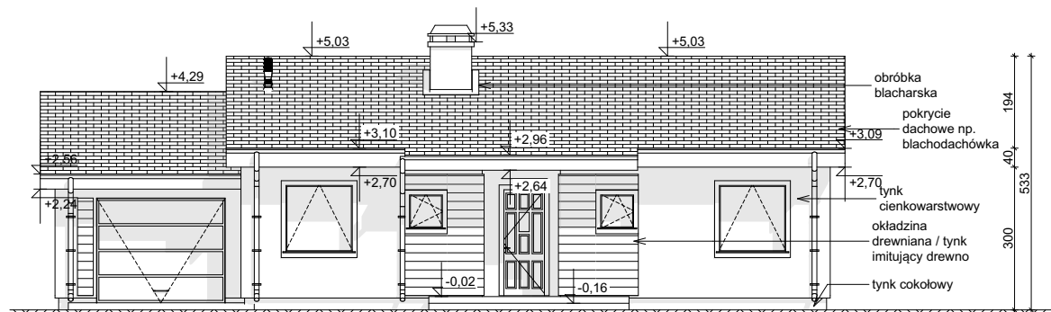
ELEWACJA FRONTOWA
