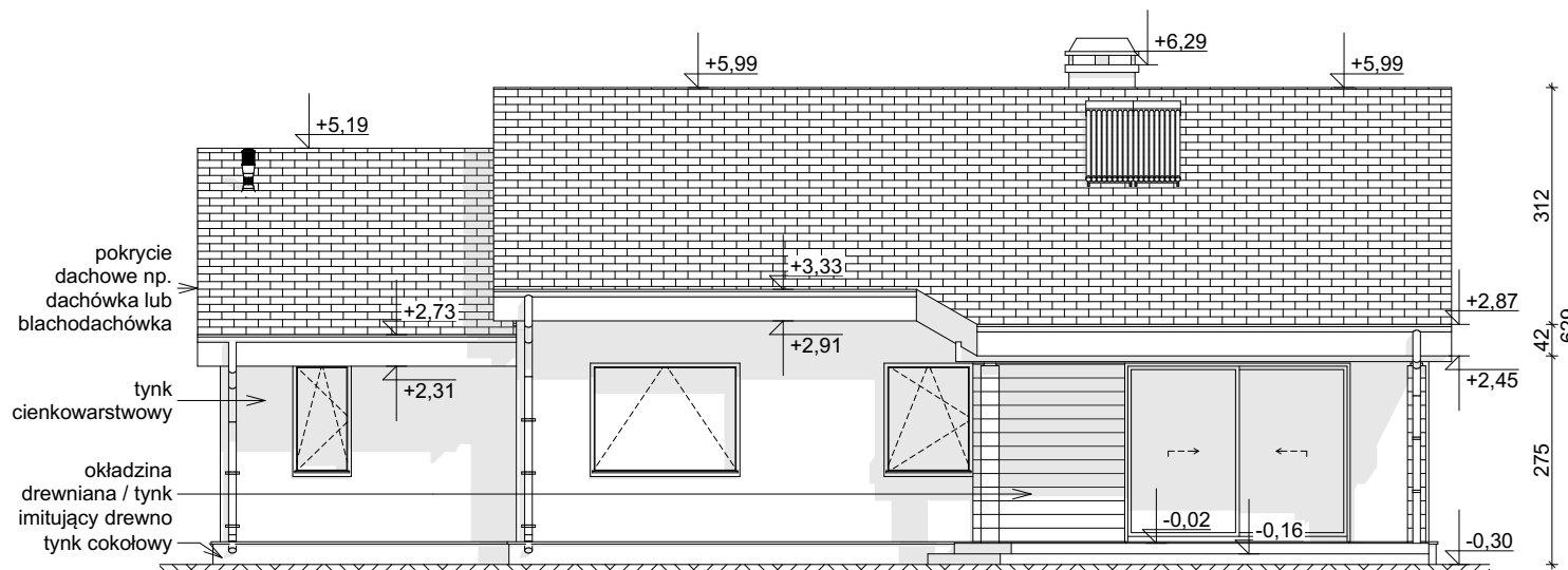
ELEWACJA OGRODOWA
