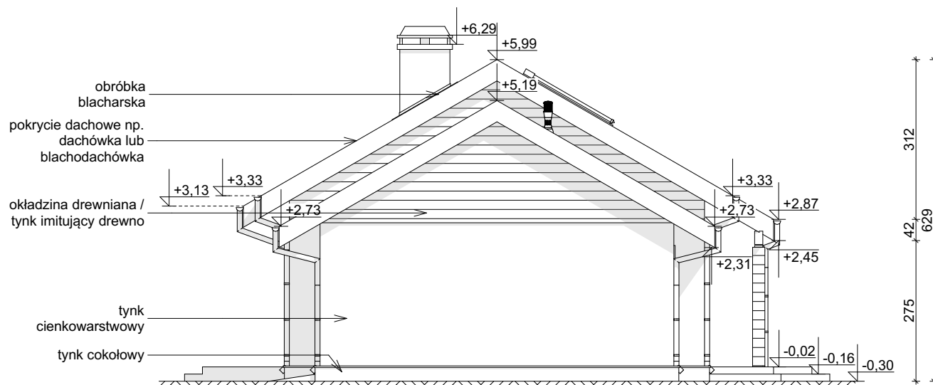
ELEWACJA BOCZNA
