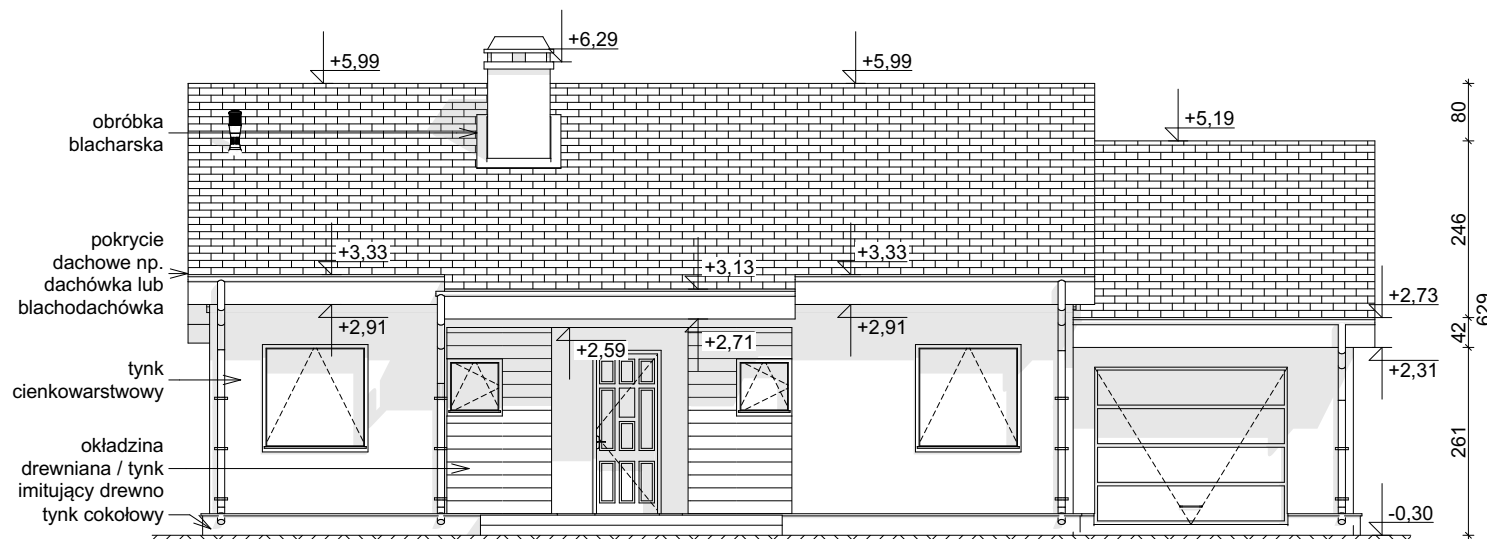
ELEWACJA FRONTOWA
