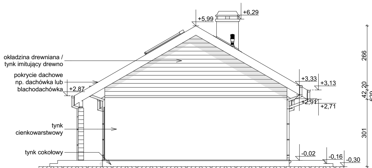
ELEWACJA BOCZNA
