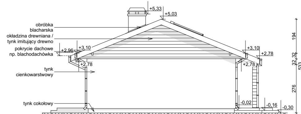
ELEWACJA BOCZNA
