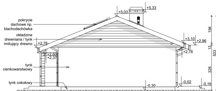
ELEWACJA BOCZNA
