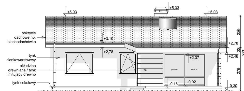
ELEWACJA OGRODOWA
