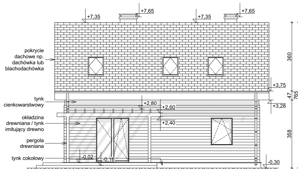
ELEWACJA OGRODOWA
