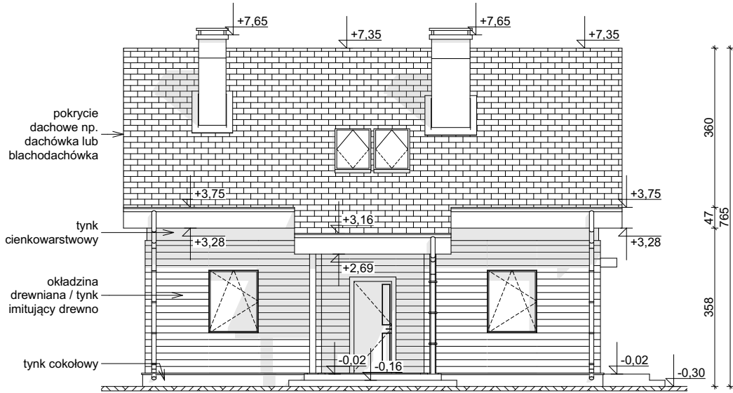
ELEWACJA FRONTOWA
