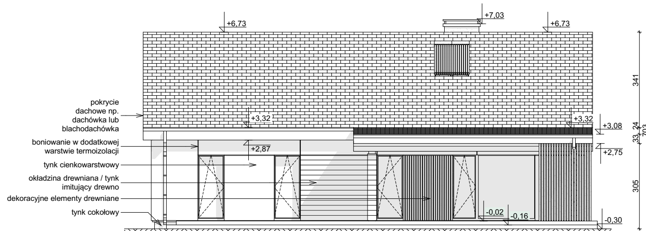
ELEWACJA OGRODOWA
