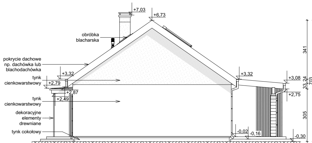
ELEWACJA BOCZNA
