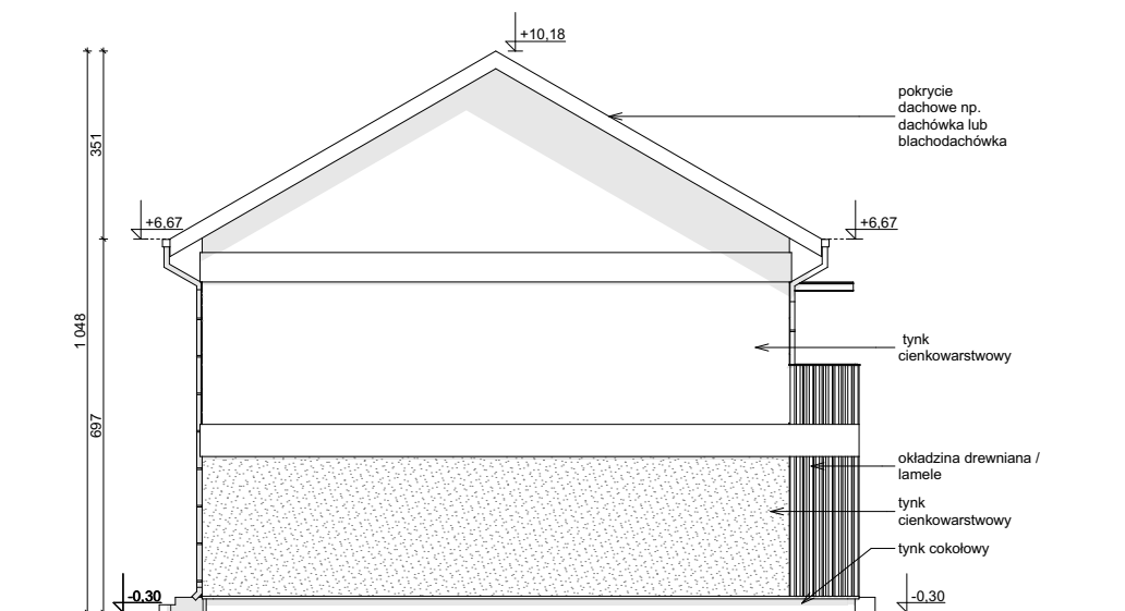
ELEWACJA BOCZNA
