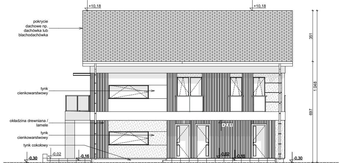
ELEWACJA FRONTOWA
