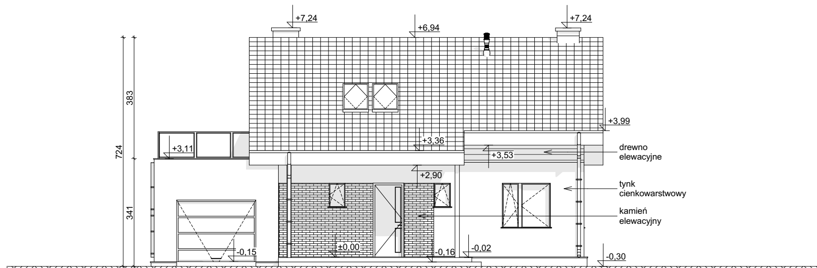
ELEWACJA FRONTOWA
