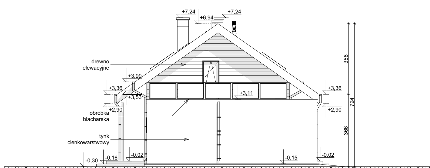
ELEWACJA BOCZNA
