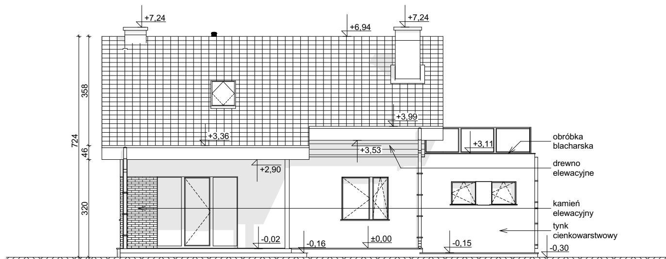
ELEWACJA OGRODOWA
