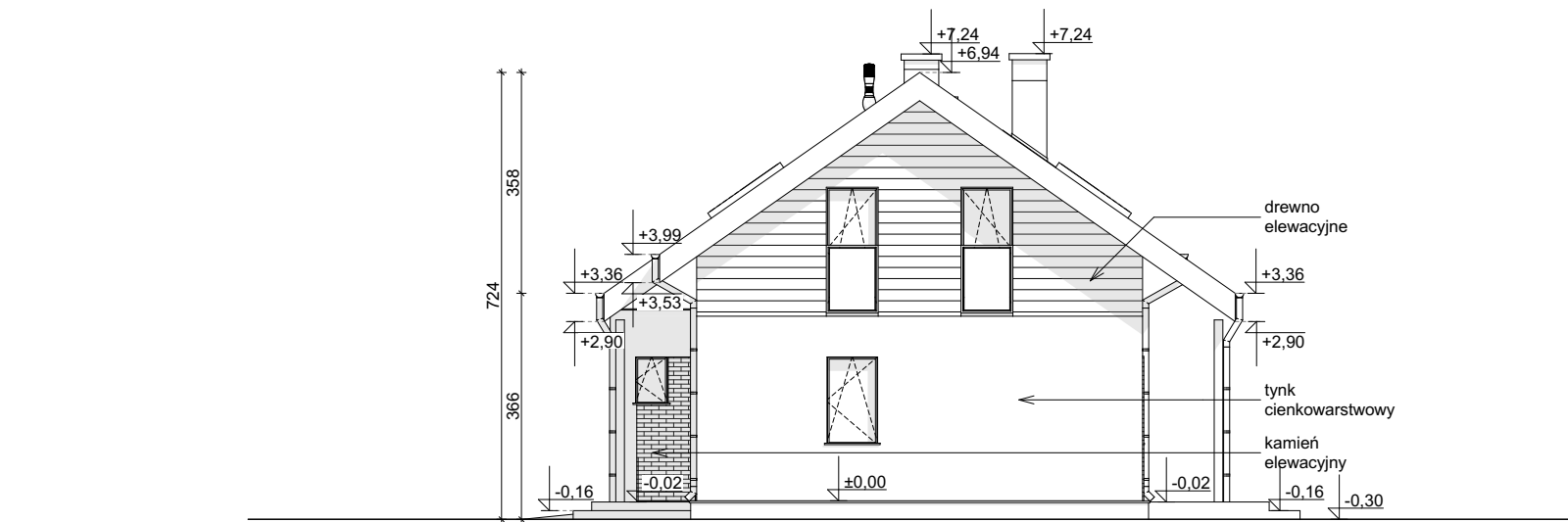
ELEWACJA BOCZNA
