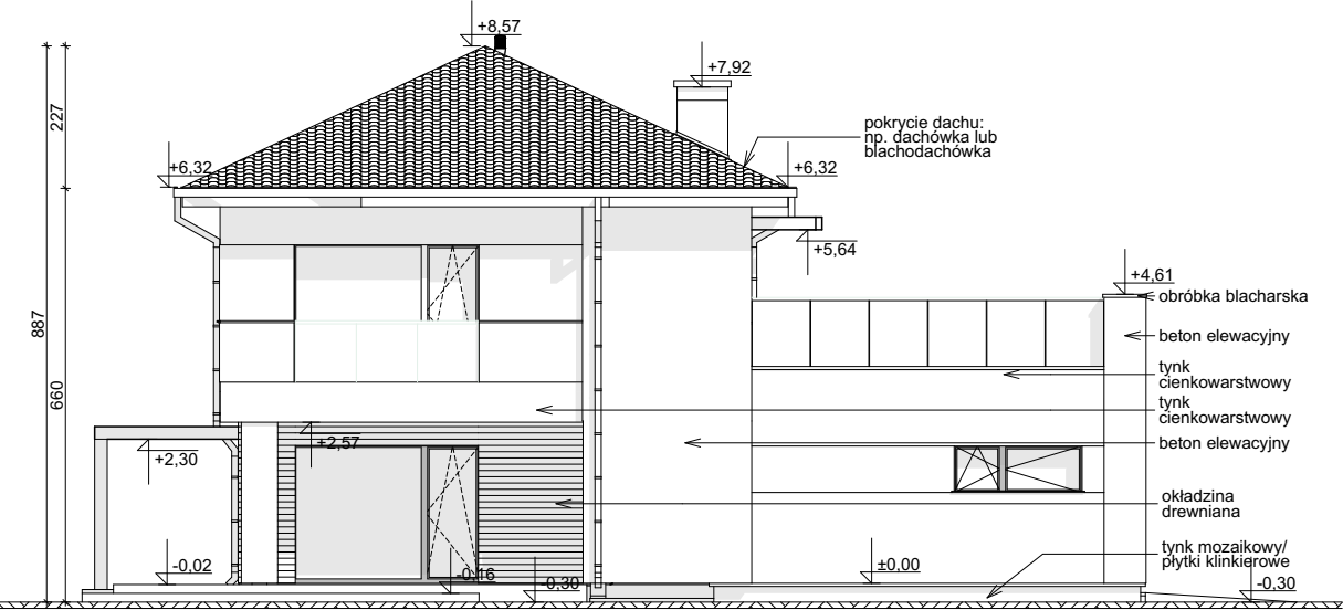
ELEWACJA OGRODOWA
