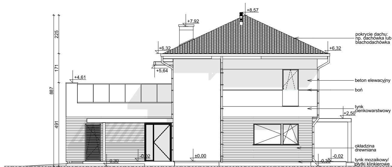
ELEWACJA FRONTOWA
