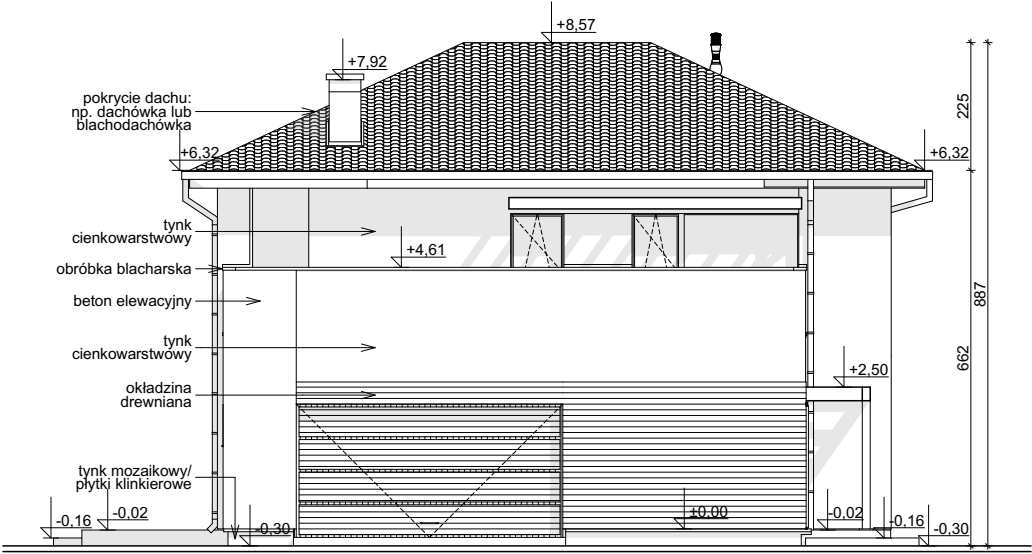
ELEWACJA BOCZNA
