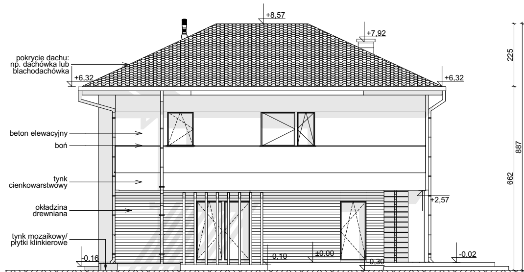
ELEWACJA BOCZNA
