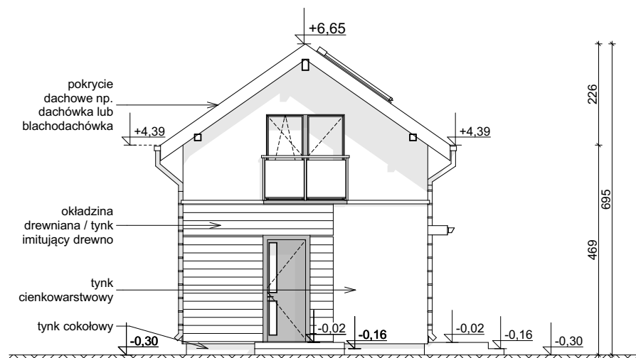
ELEWACJA FRONTOWA
