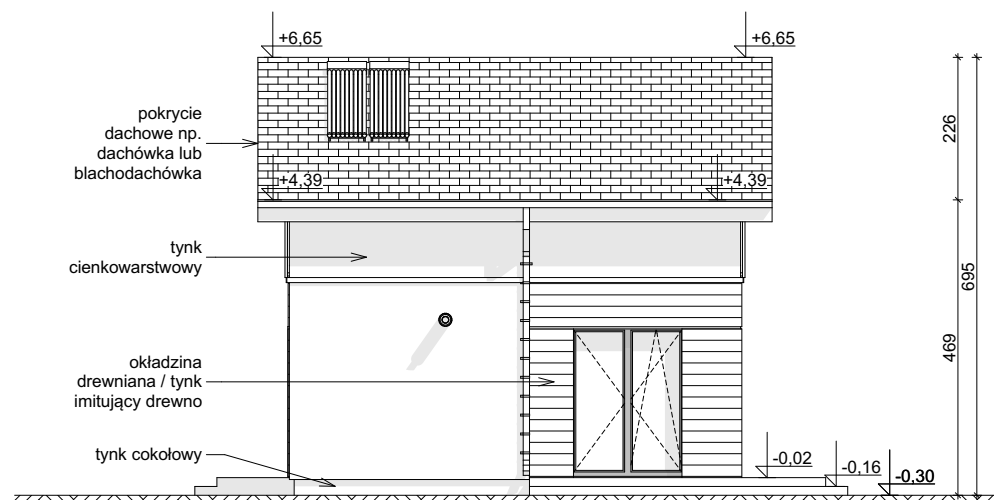
ELEWACJA BOCZNA
