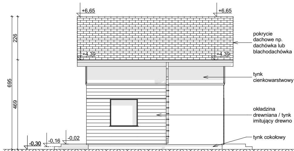
ELEWACJA BOCZNA
