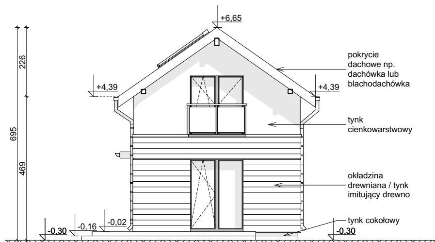
ELEWACJA OGRODOWA
