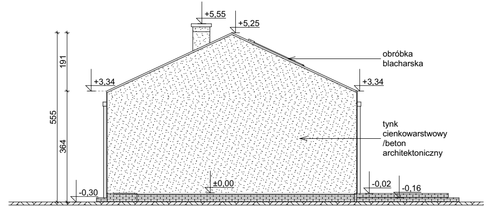
ELEWACJA BOCZNA
