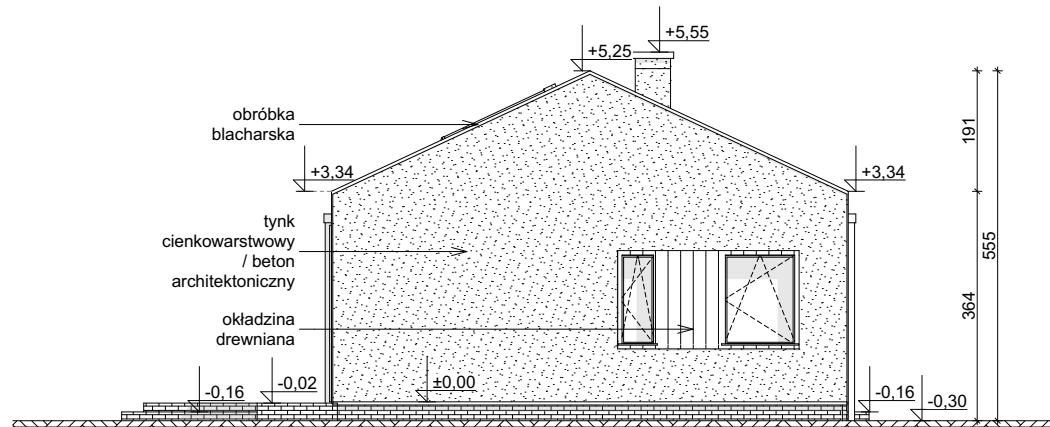
ELEWACJA BOCZNA
