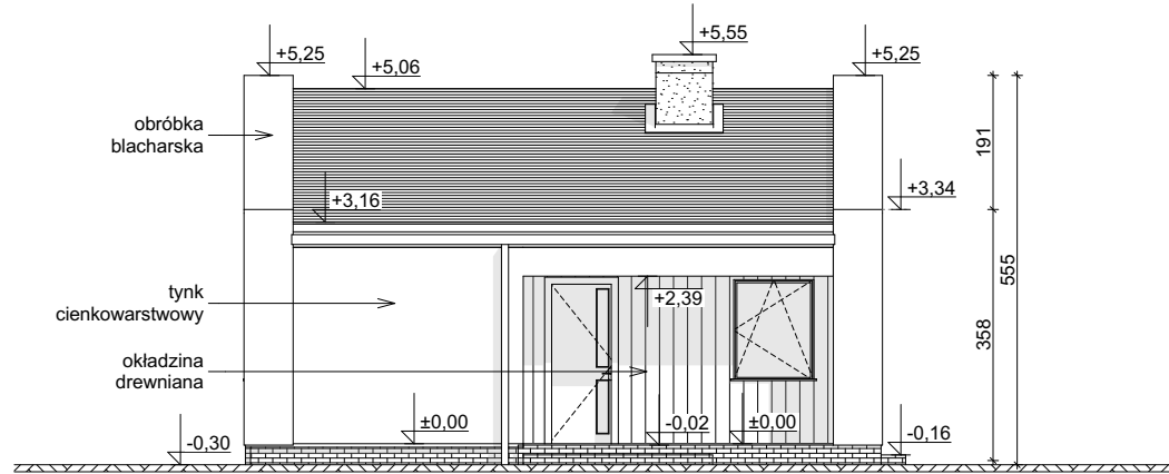
ELEWACJA FRONTOWA
