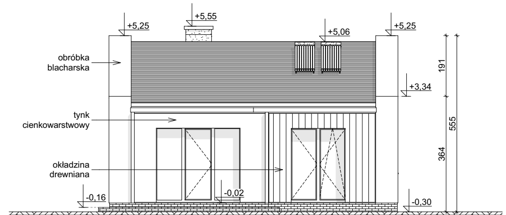
ELEWACJA OGRODOWA
