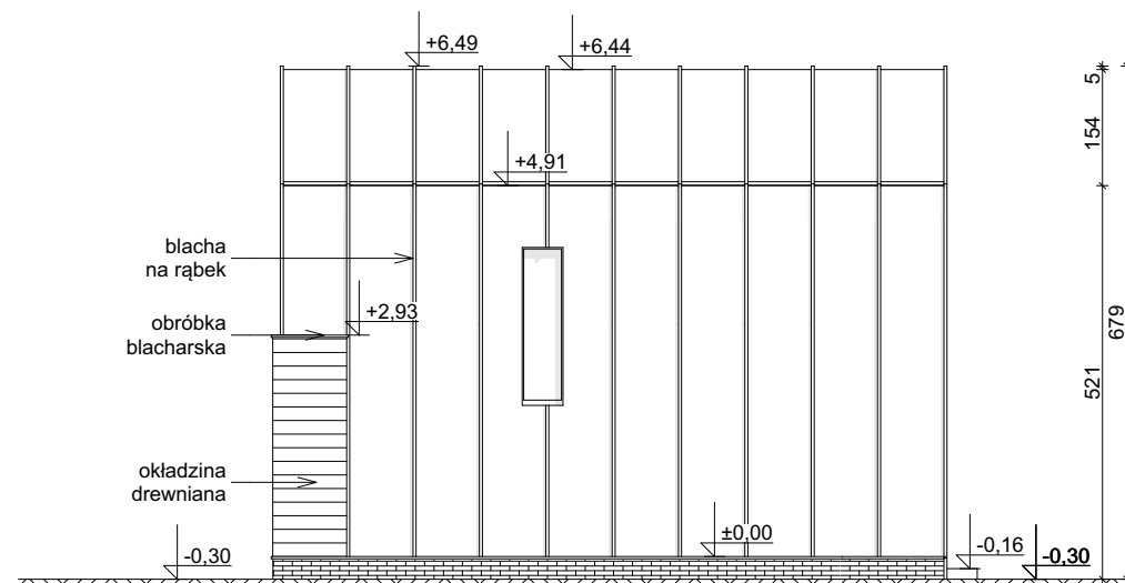
ELEWACJA OGRODOWA
