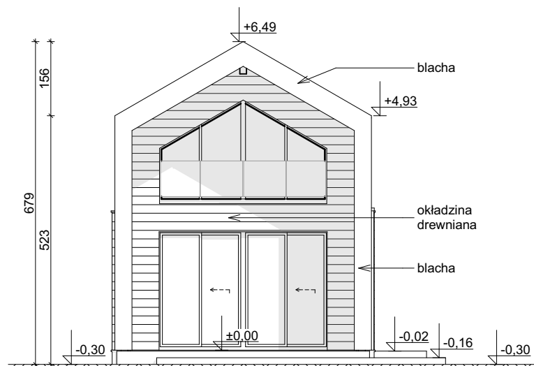
ELEWACJA BOCZNA
