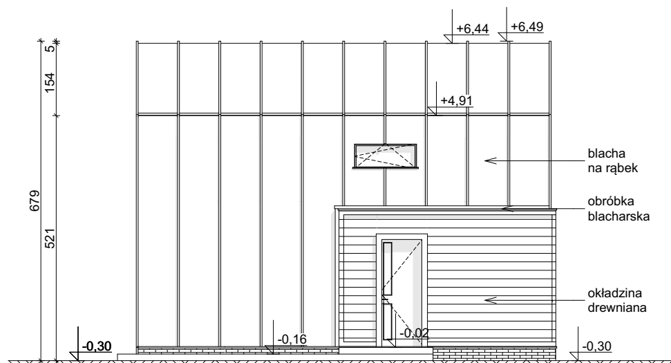
ELEWACJA FRONTOWA
