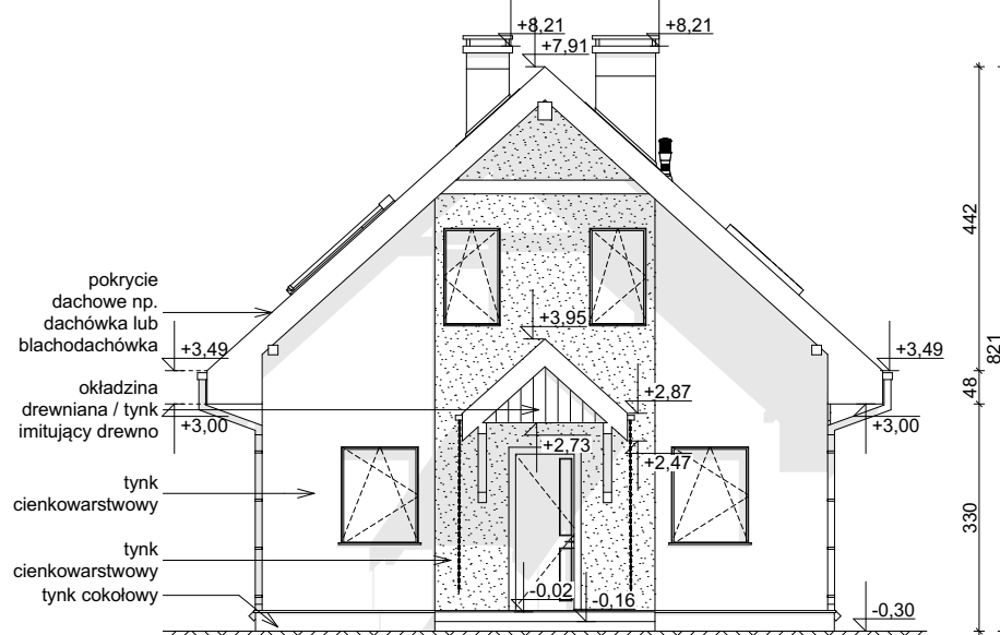
ELEWACJA FRONTOWA
