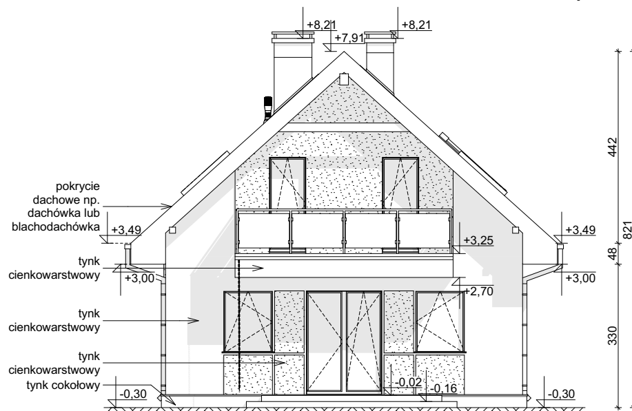
ELEWACJA OGRODOWA
