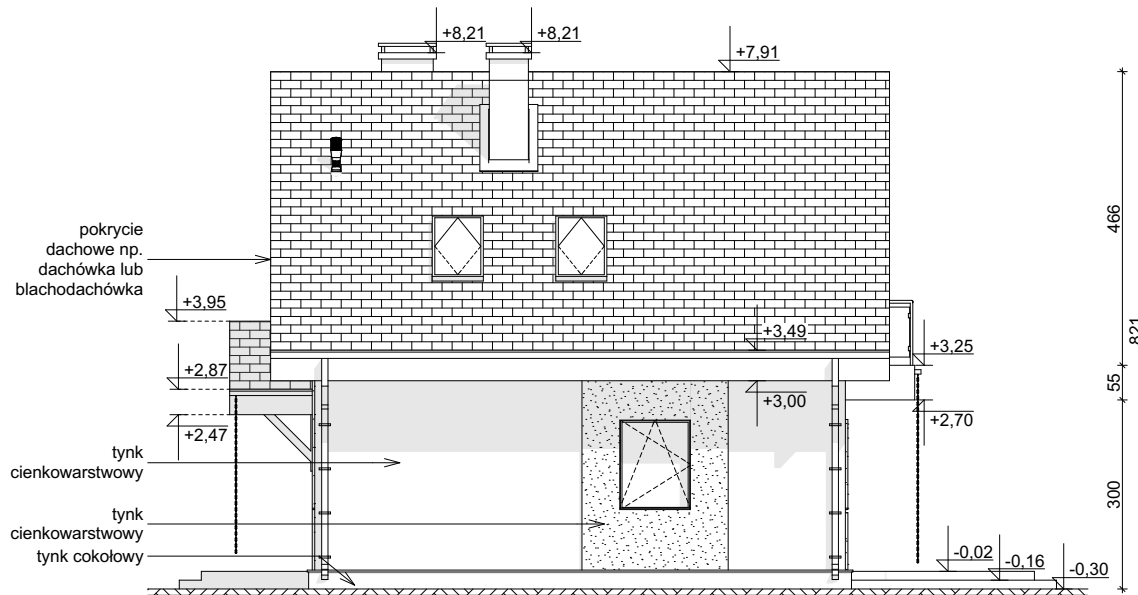
ELEWACJA BOCZNA
