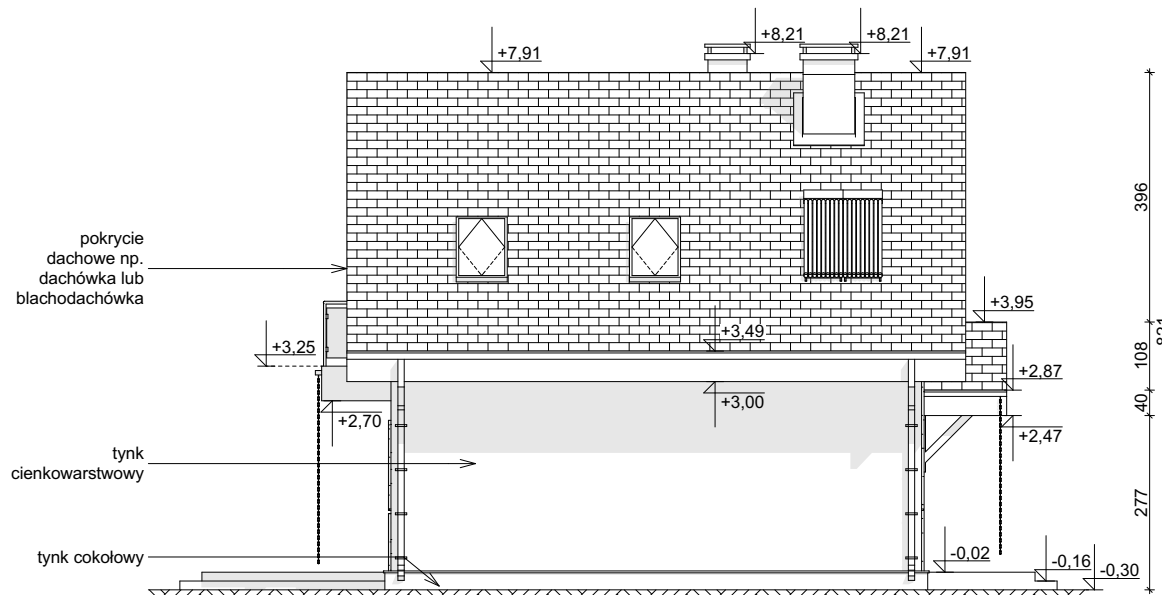
ELEWACJA BOCZNA
