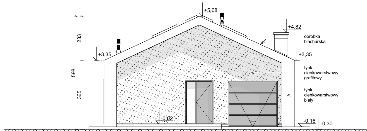
ELEWACJA FRONTOWA
