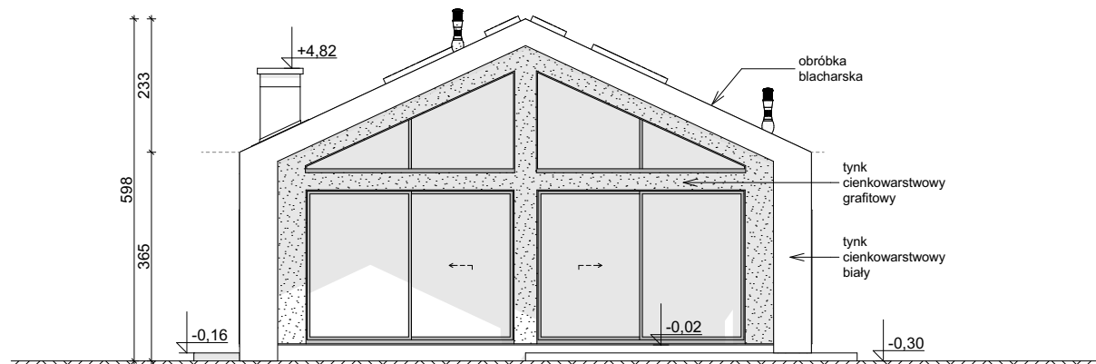
ELEWACJA OGRODOWA
