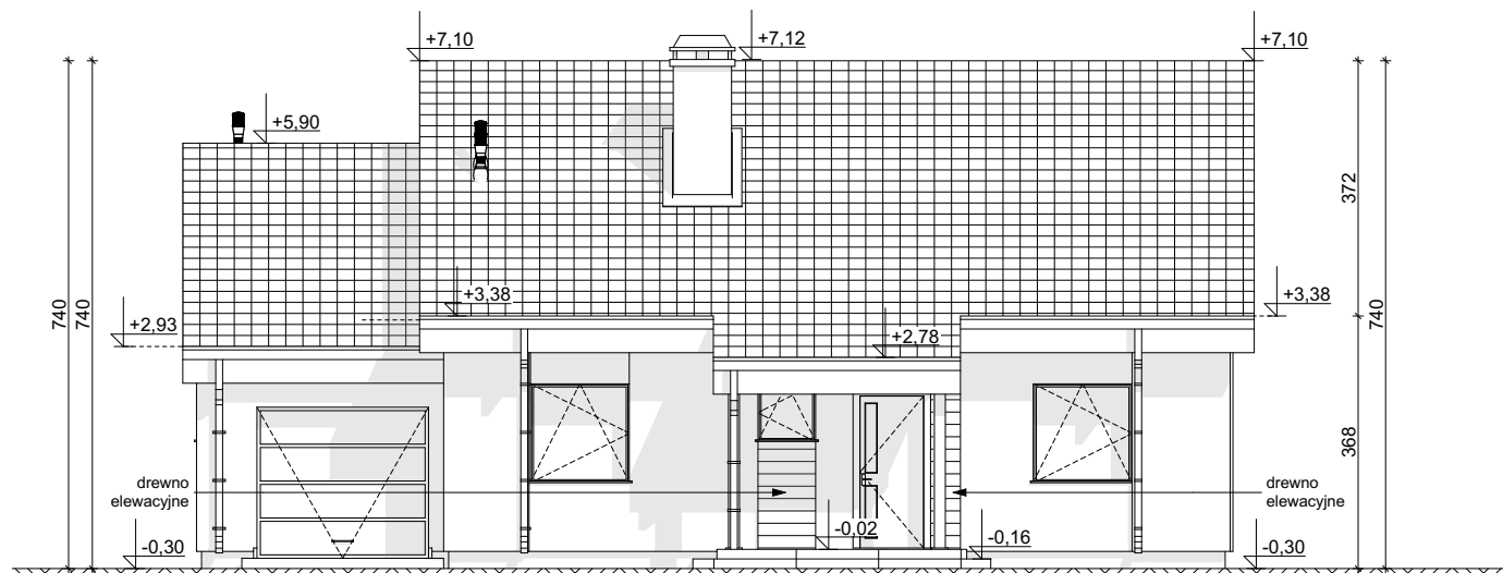
ELEWACJA FRONTOWA
