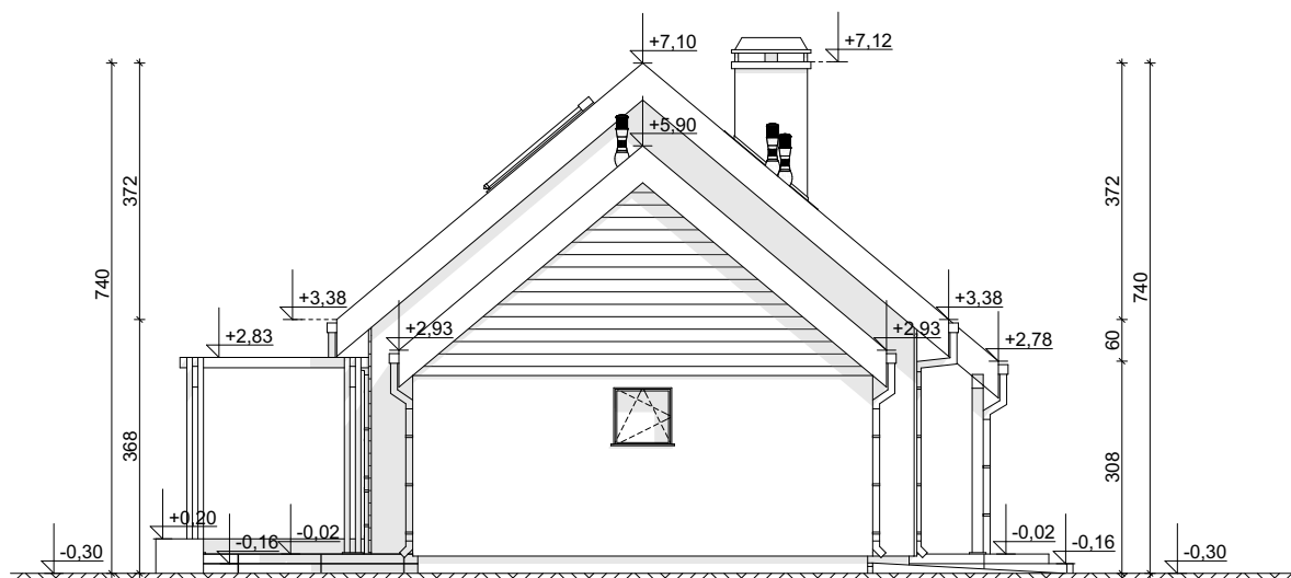
ELEWACJA BOCZNA
