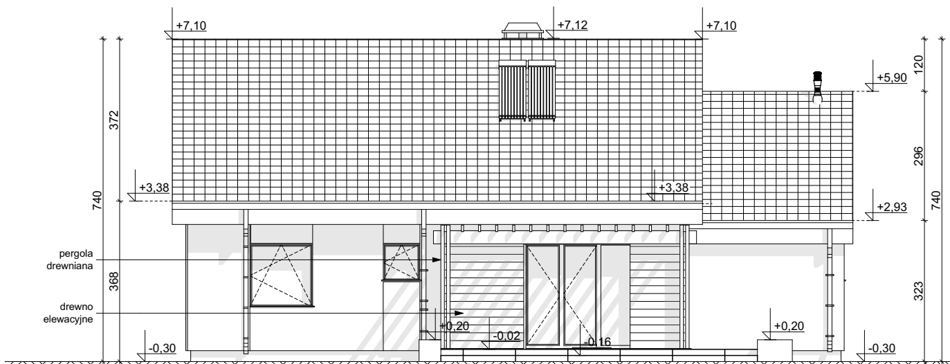
ELEVACJA OGRODOWA
