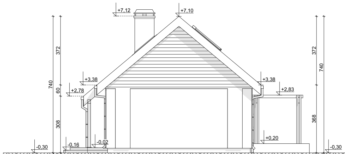
ELEVACJA BOCZNA
