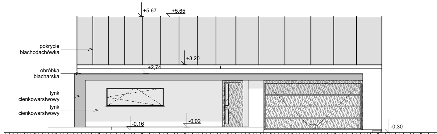
ELEWACJA FRONTOWA
