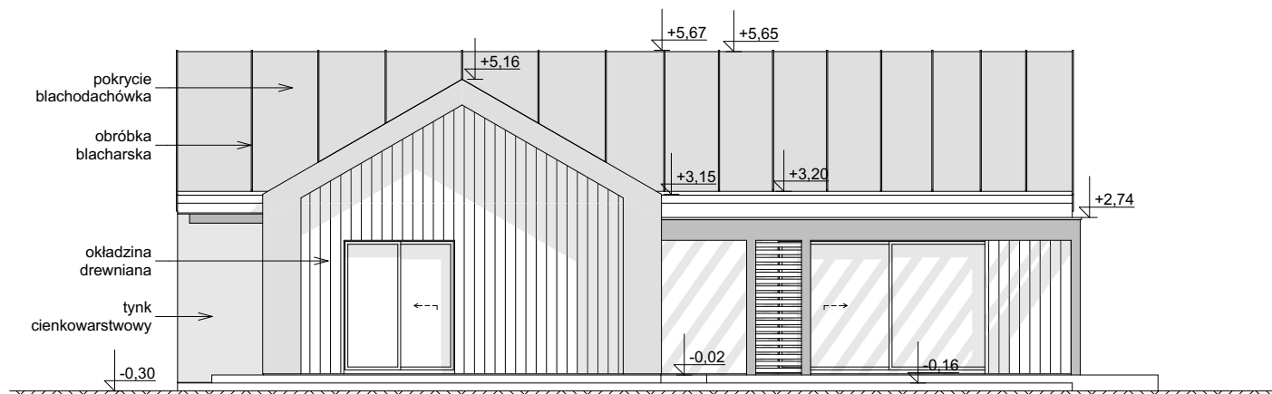
ELEWACJA OGRODOWA
