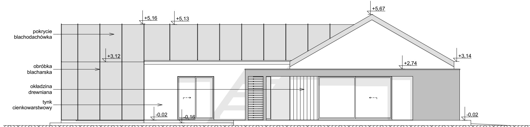
ELEWACJA BOCZNA
