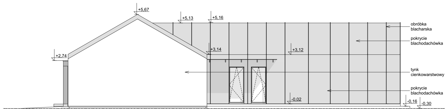
ELEWACJA BOCZNA
