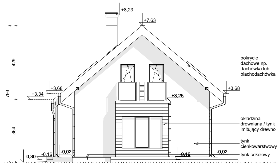
ELEWACJA BOCZNA
