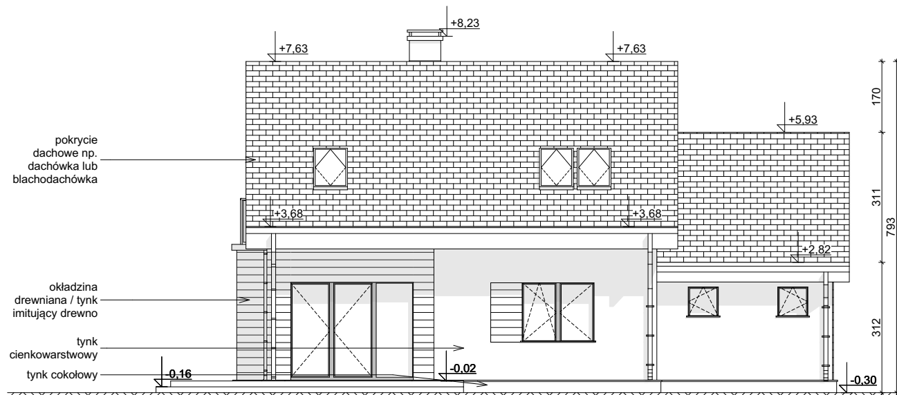
ELEWACJA OGRODOWA
