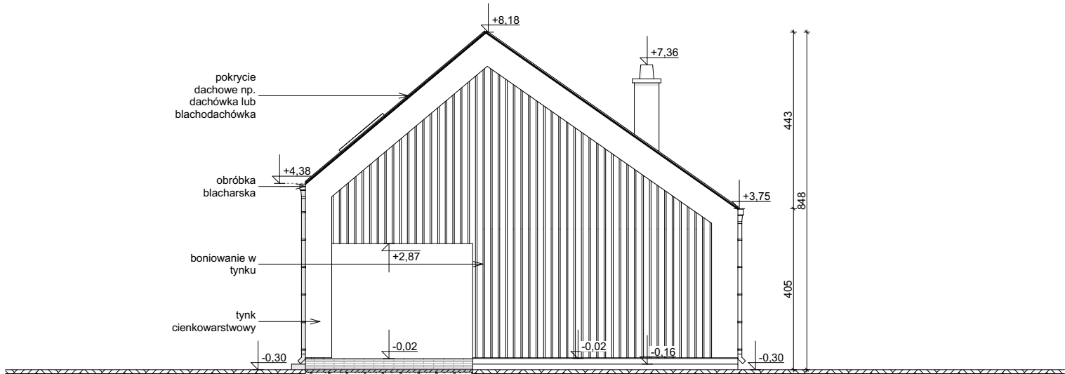
ELEWACJA FRONTOWA
