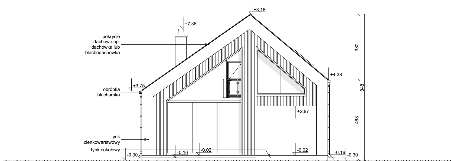
ELEWACJA OGRODOWA
