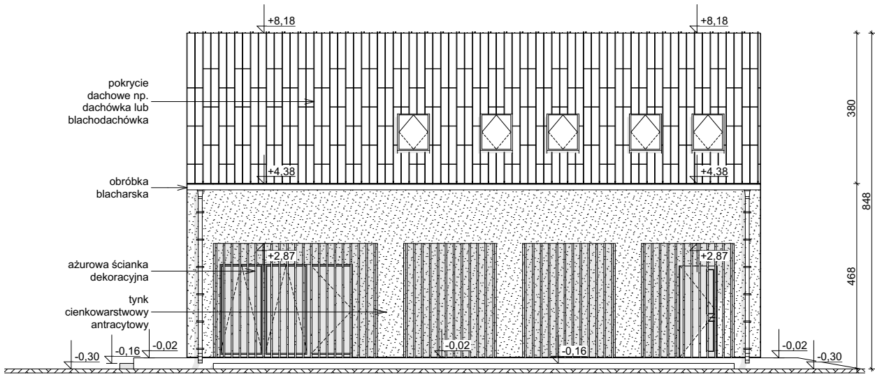
ELEWACJA BOCZNA
